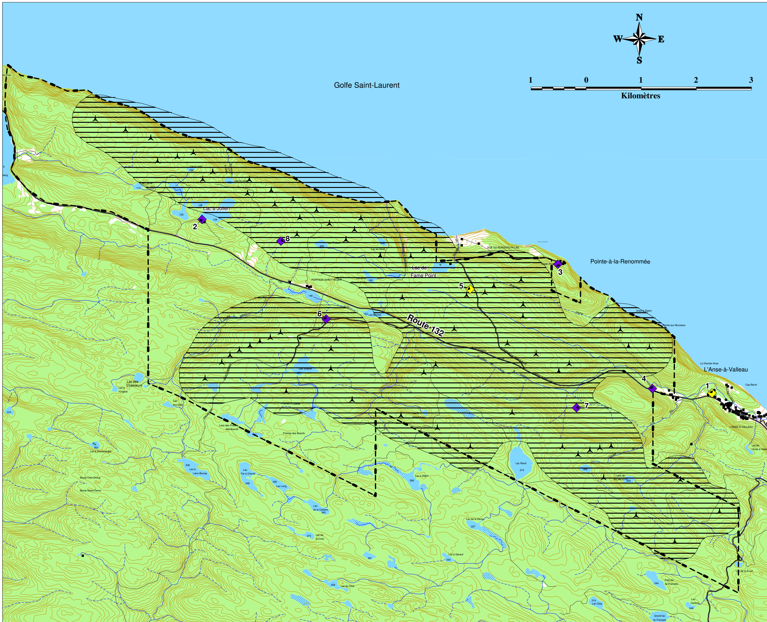
Carte 5.3 Contour isophonique du parc éolien (42 dBA)
