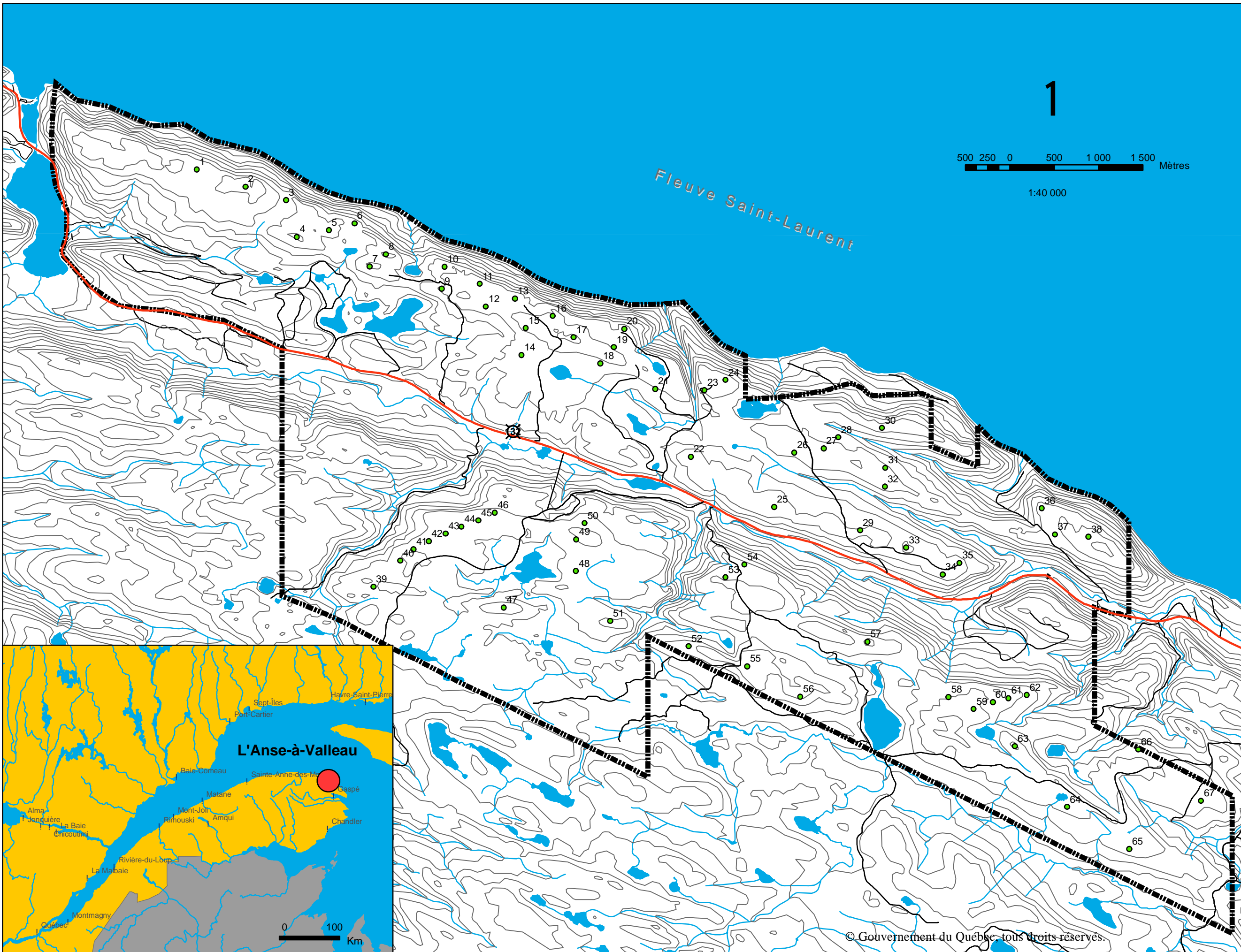
Carte 2.2 Positionnement des éoliennes dans le domaine du parc
