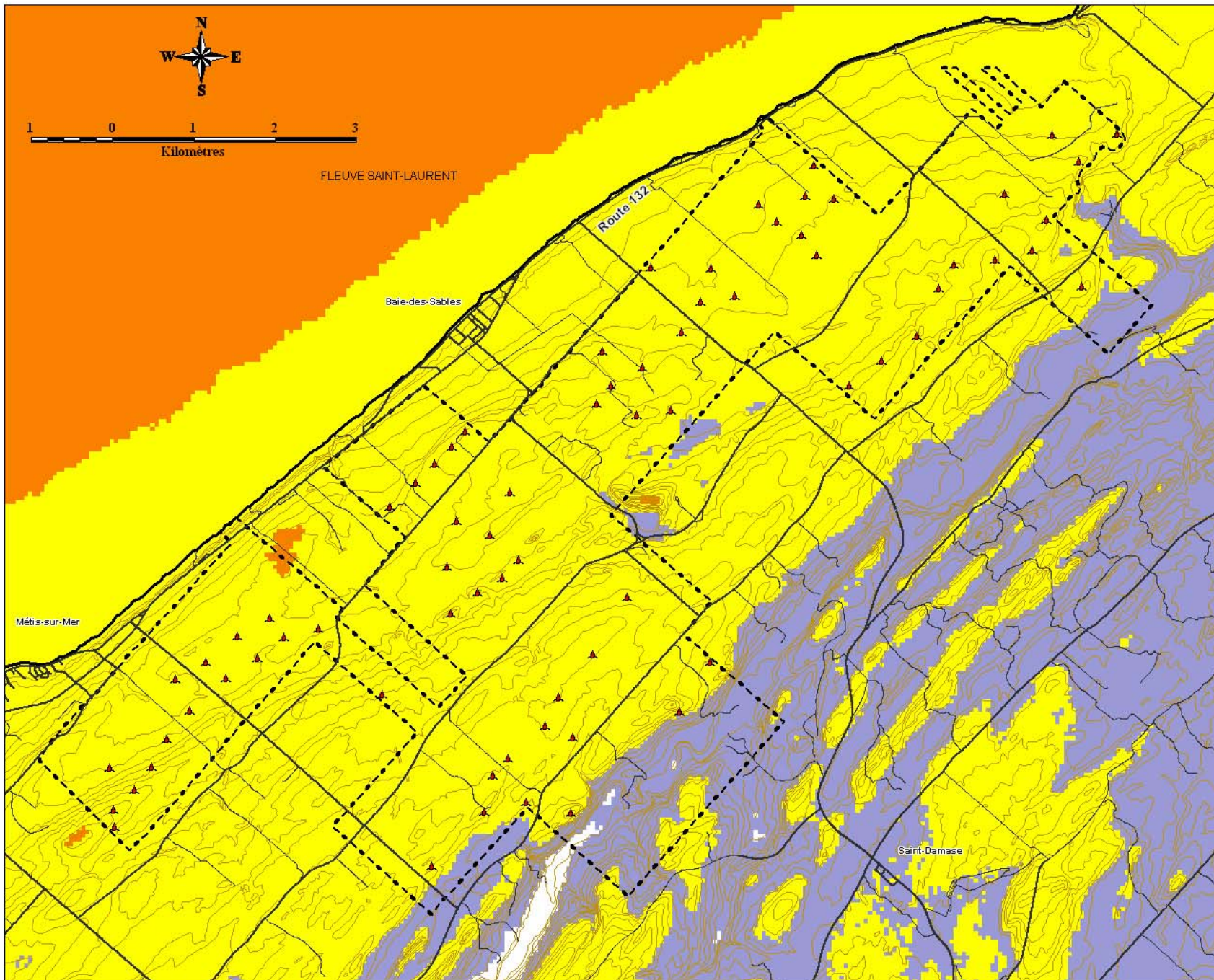
Carte 3.2 Qualité du gisement éolien (Mars 2005)
