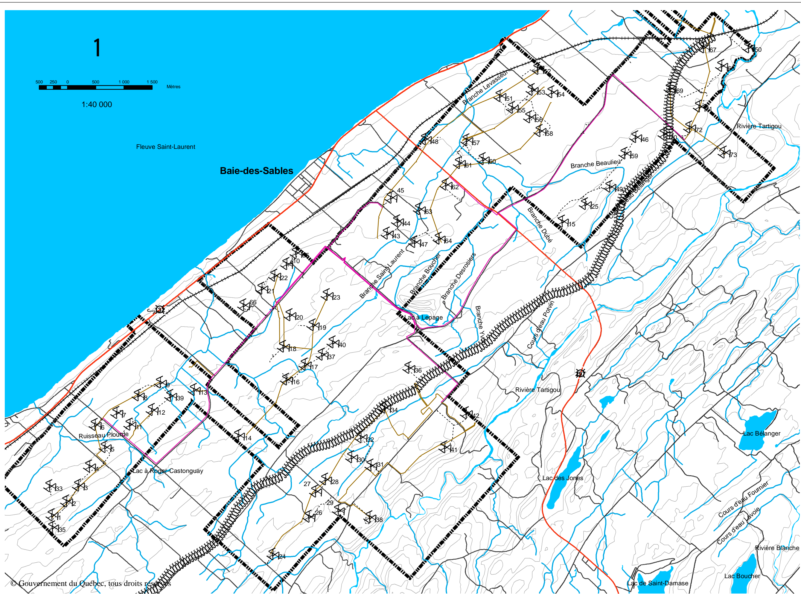
Carte 2.4 Réseau hydrographique du secteur de Baie-des-Sables (31 mars 2005)
