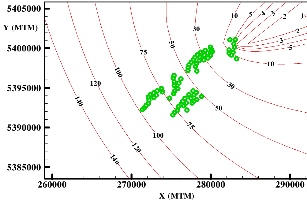
Figure 3. Carte du délai maximum (en \mu\text{s} )
