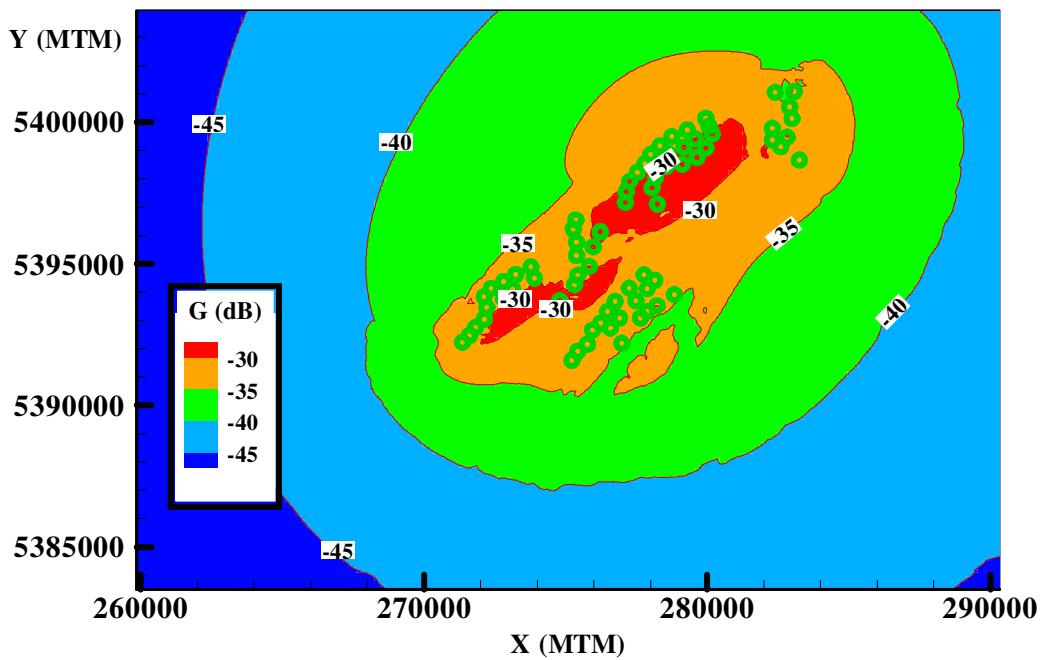
Figure 4. Carte du rapport d'écho G (dB)
