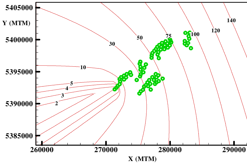
Figure 1. Carte du délai maximum (en \mu\text{s} )
