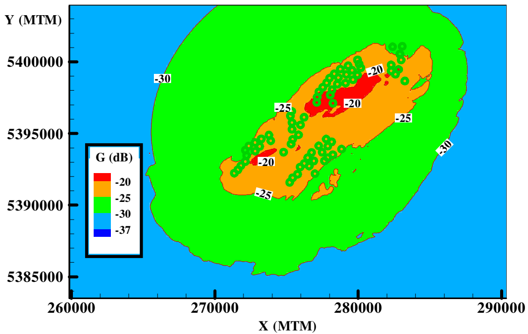
Figure 2. Carte du rapport d'écho G (dB)
