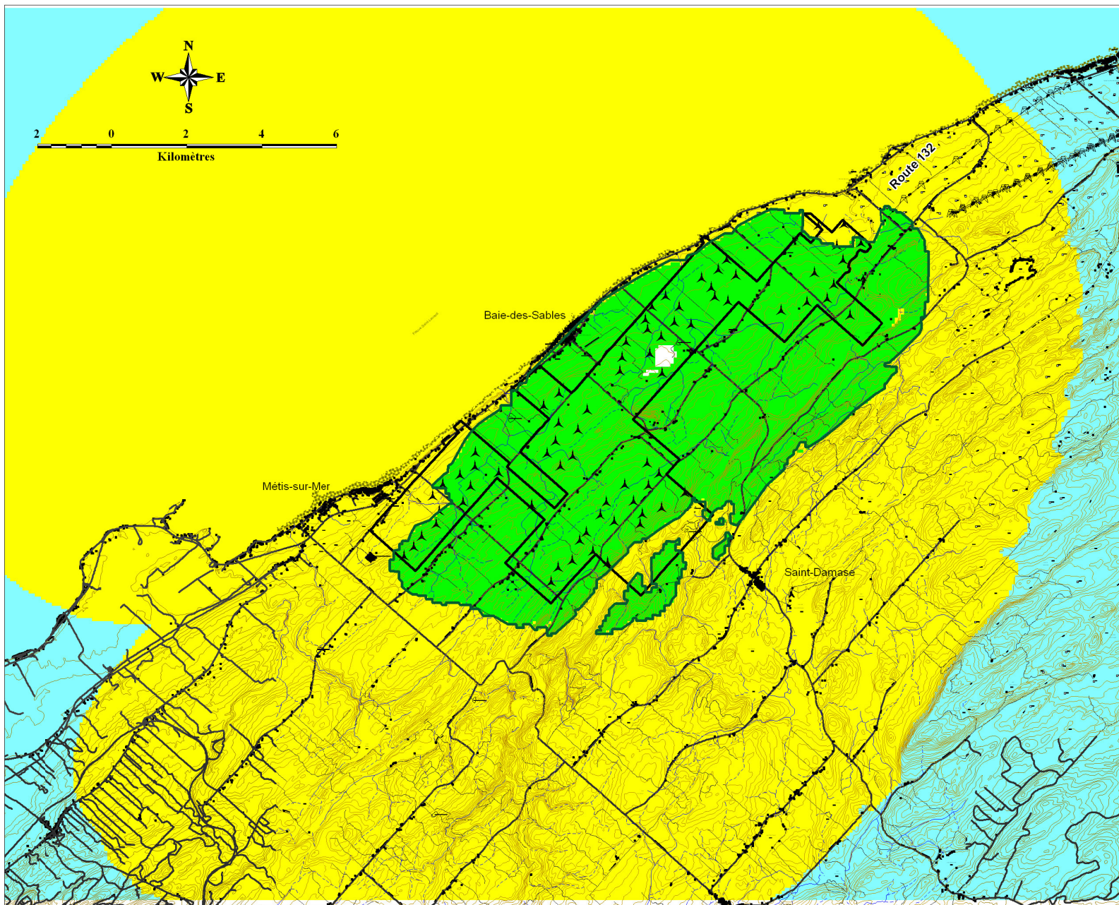
Carte 2 Prévision du brouillage par fantômes (CBGAT-TV)
