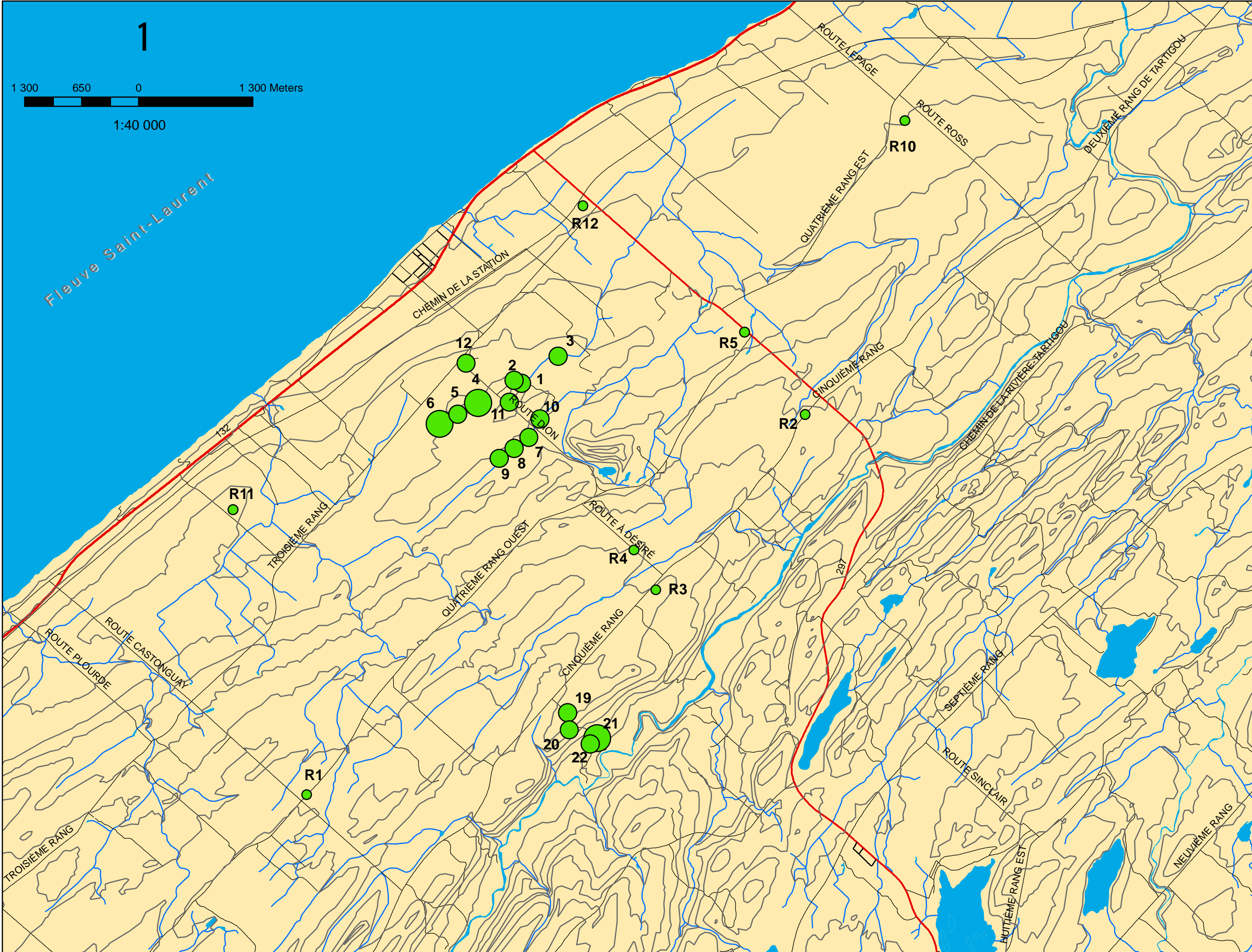
Carte 9. Diversité relative des oiseaux observés lors de l'inventaire ornithologique automnal réalisé dans le secteur de Baie-des-Sables
