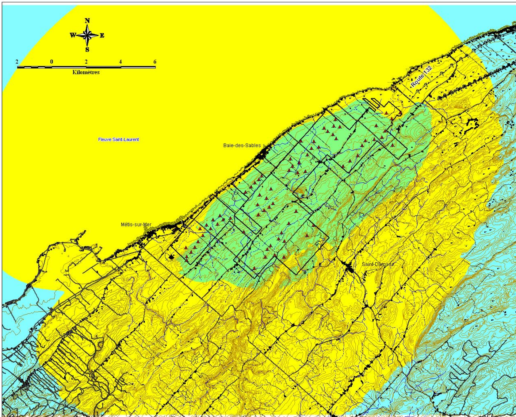
Carte 2 Prévision du brouillage par fantômes (CBGAT-TV) (Mars 2005)
