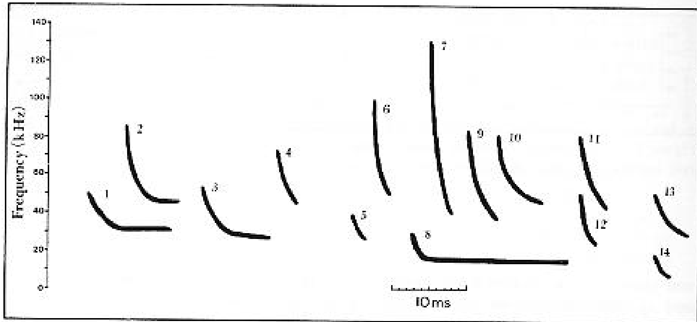
Figure 9. Sound spectrograms of the fundamental search phase echolocation calls of Canadian bats showing frequency change over time. 1) L. cinereus ; 2) M. volans ; 3) E. fuscus ; 4) P. subflavus ; 5) P. townsendii ; 6) M. evotis ; 7) M. septentrionalis ; 8) T. macrotis ; 9) M. lucifigus ; 10) M. ciliolabrum ; 11) M. californicus ; 12) A. pallidus ; 13) M. thysanodes ; 14) E. maculatum .
