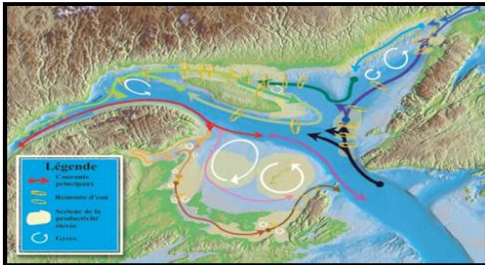
Figure 9 Courants marins dans le golfe du Saint-Laurent
