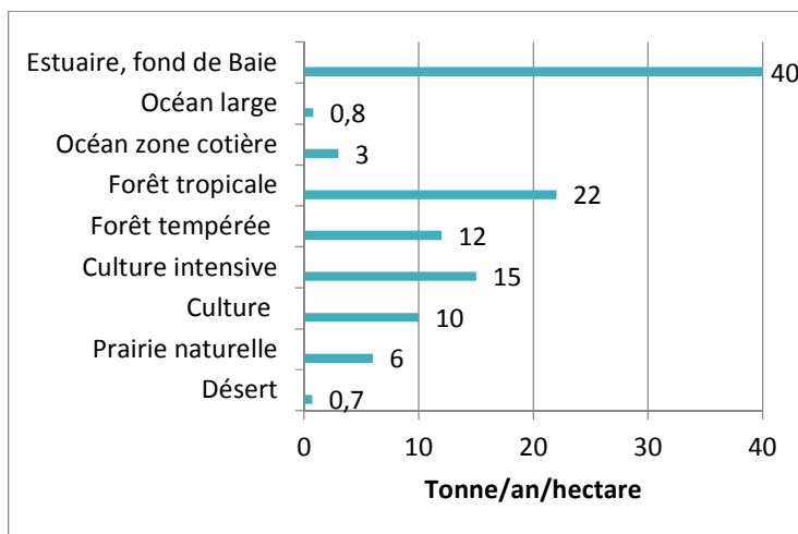
Figure 7 Milieux naturels les plus productifs au monde en matière organique par hectare
