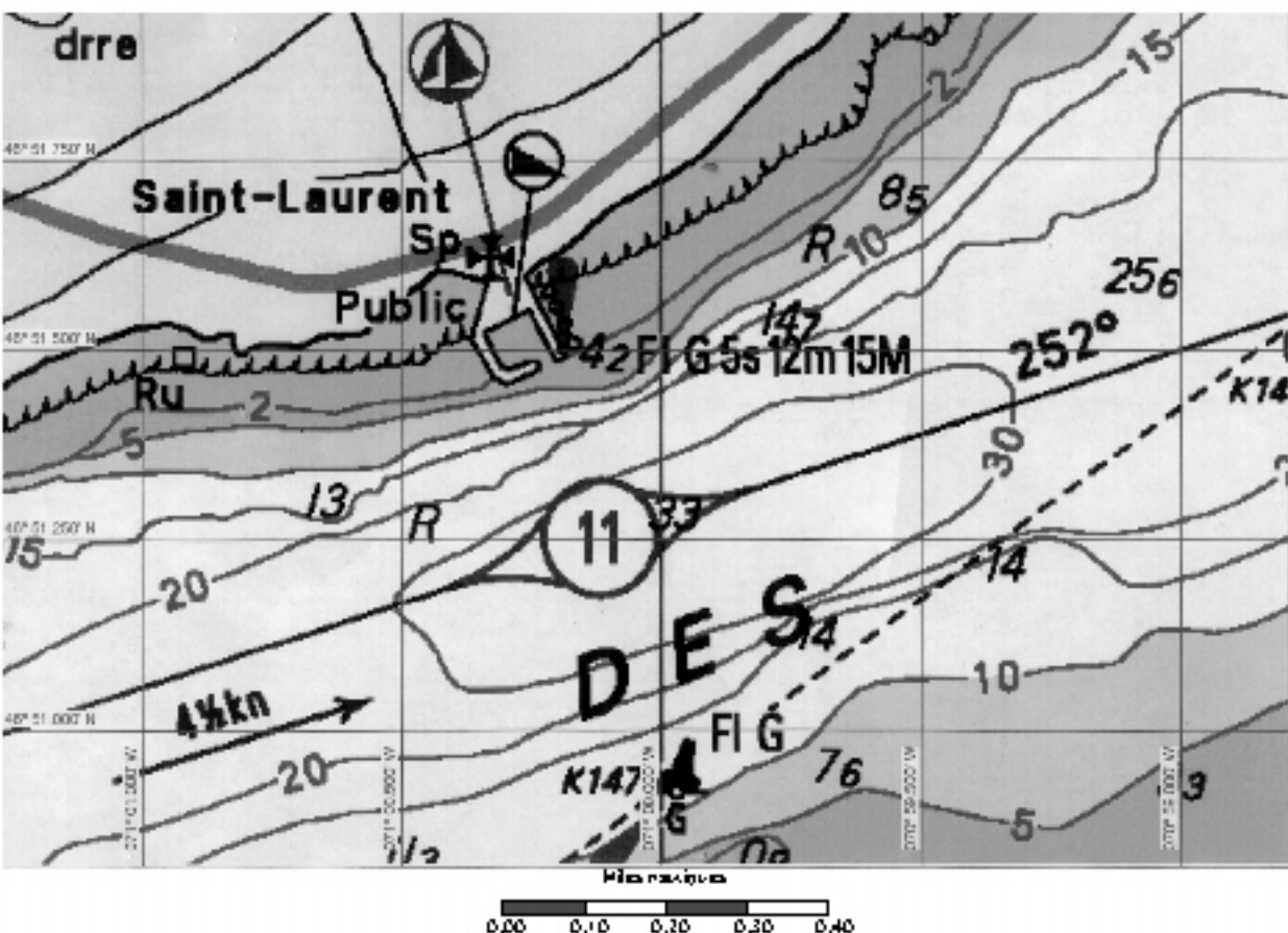
Figure 4: Description de la bathymétrie en avant du quai de Saint-Laurant à deux échelles différentes (toutes les profondeurs sont en mètres). Source: carte marine 131702
