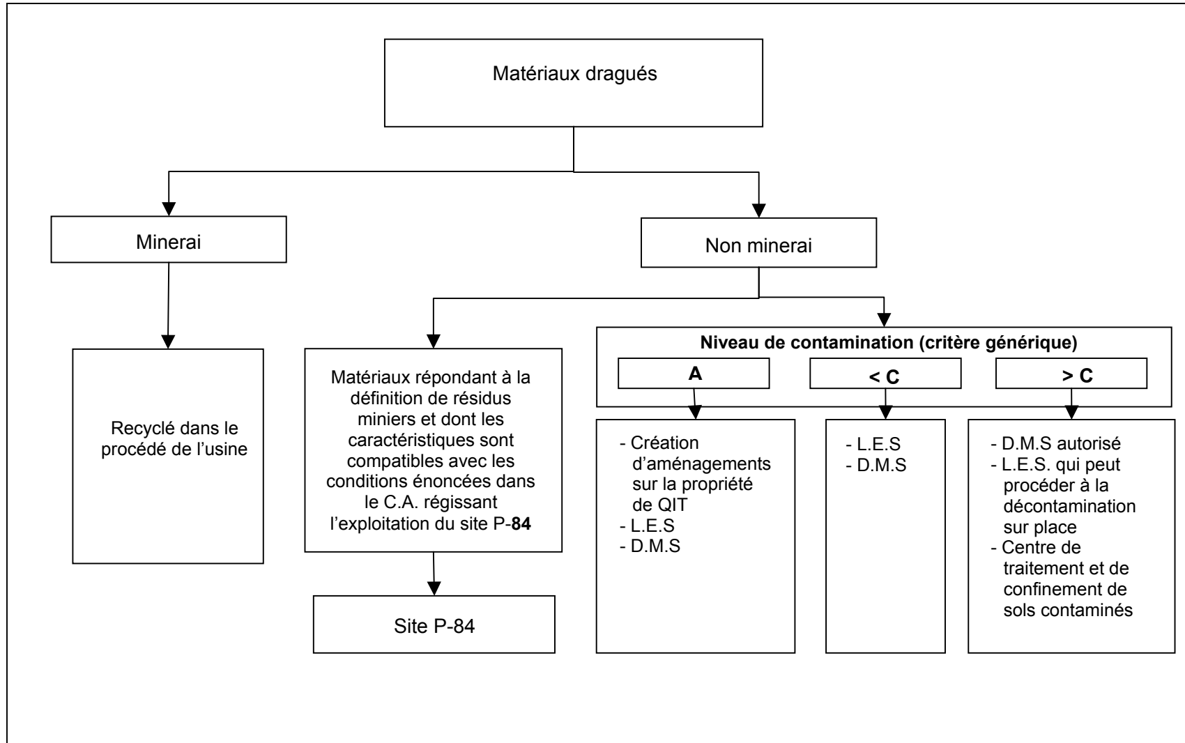
Figure 4.1 Diagramme décisionnel pour le choix du site de disposition des matériaux dragués
