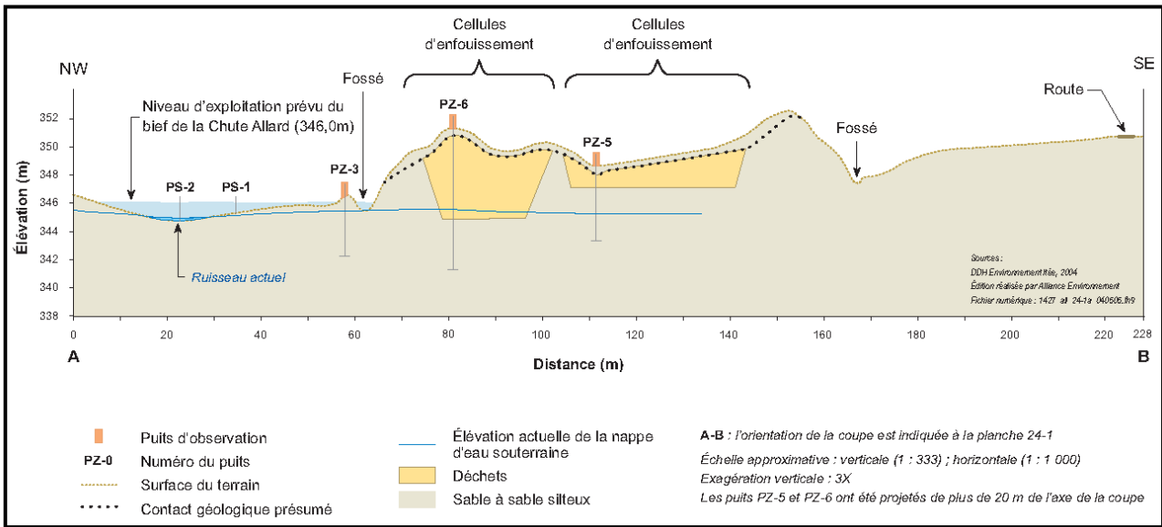
Figure 24-3 Coupe longitudinale du dépôt en tranchée de Wemotaci
