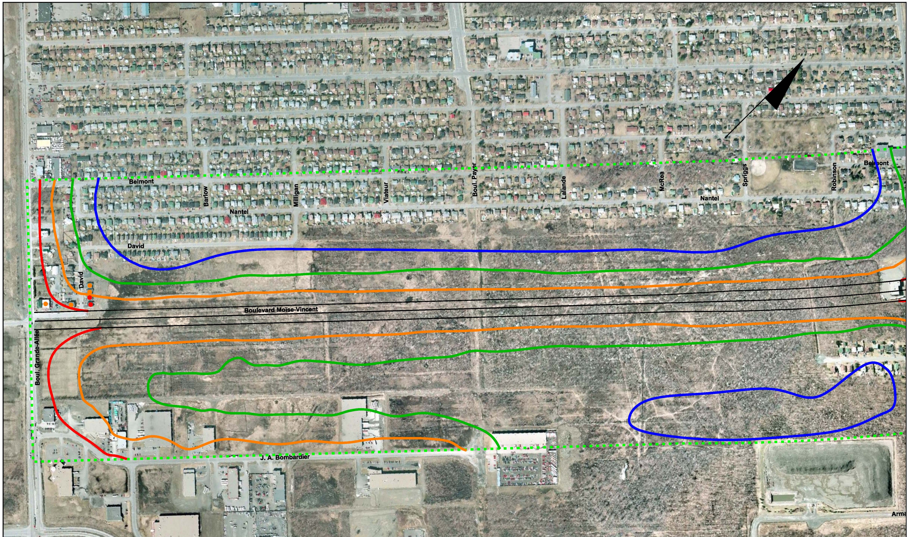
SM Aménatech Inc Figure 12 : Climat sonore projeté (2017)
