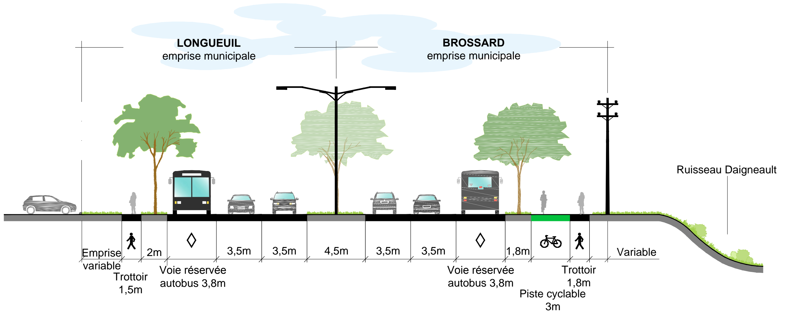
Coupe type Élargissement de la Grande-Allée
