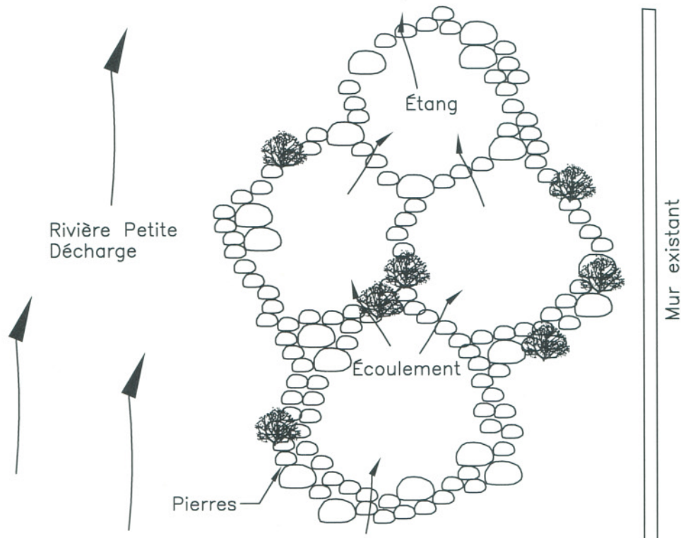
VUE EN PLAN ÉCHELLE: AUCUNE
