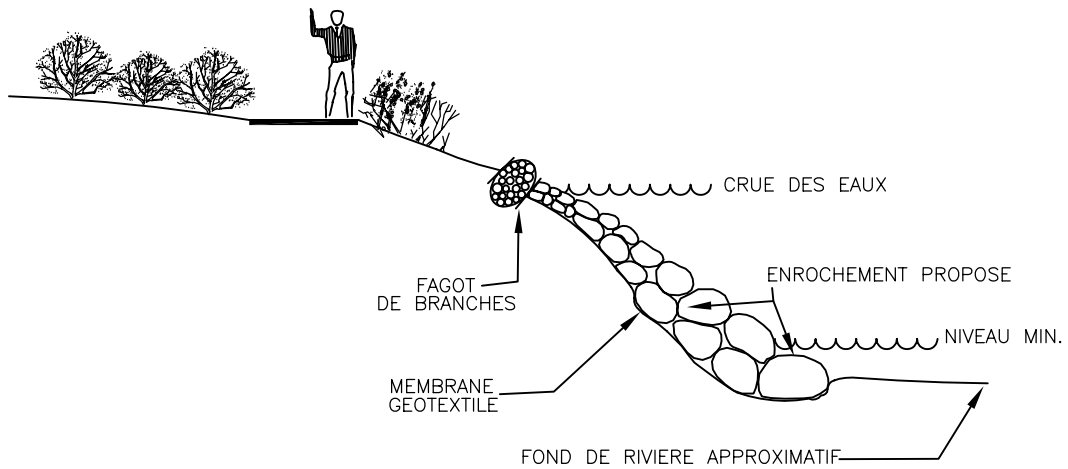
COUPE ÉCHELLE: AUCUNE
