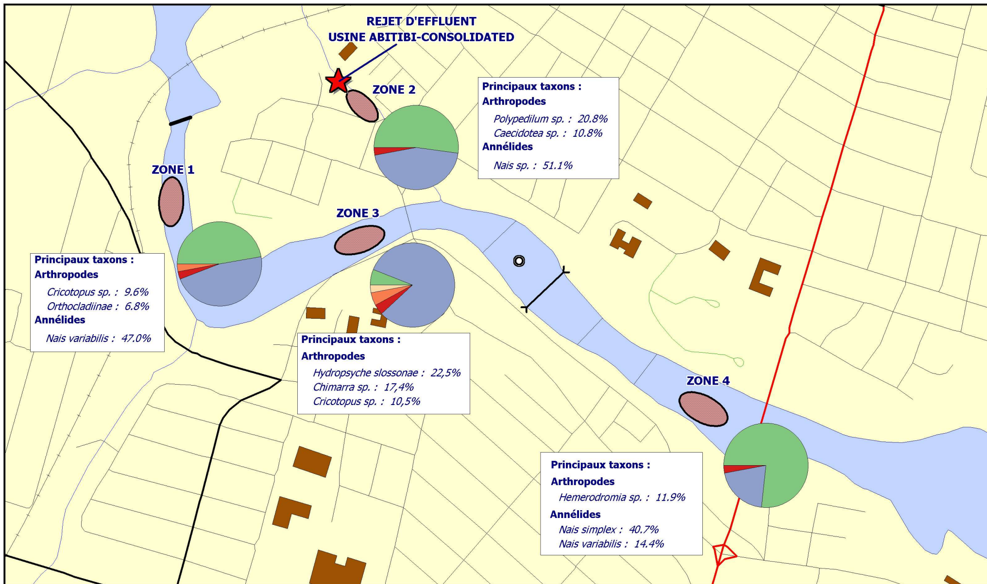
FIGURE 2.16 ZONES D'ÉCHANTILLONNAGE ET FRÉQUENCE DES INVERTÉBRÉS BENTHIQUES
