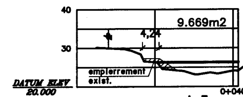
cl_5
