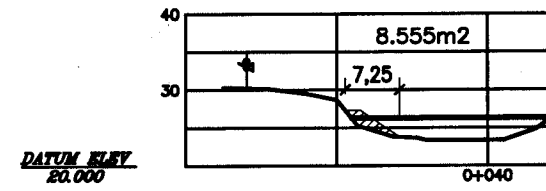
cl_1
