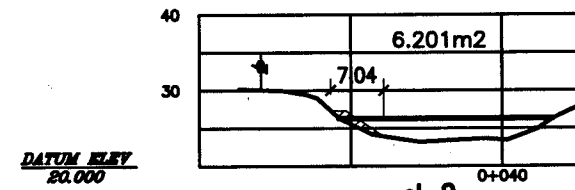
cl_2
