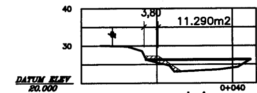
cl_4
