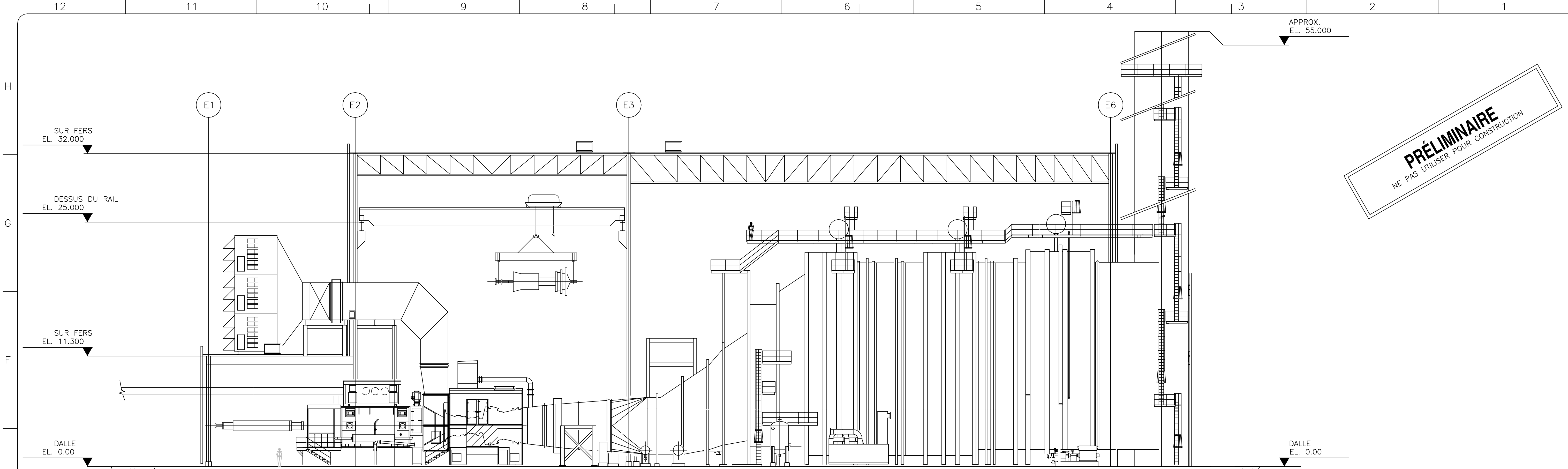
SECTION A-A ECH.: 1:200 A1-121721-1201
