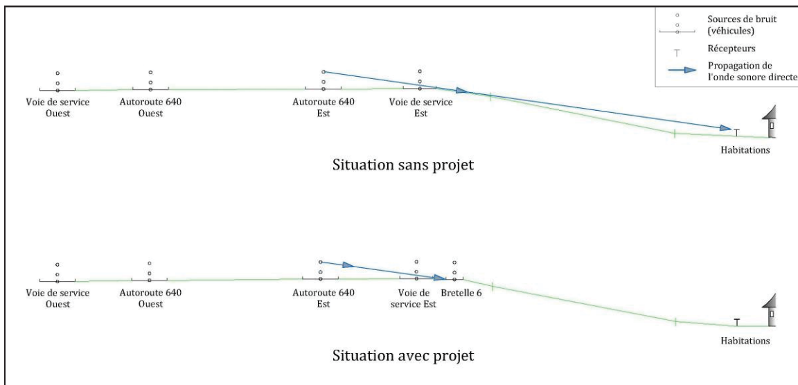
Figure 5 Coupe à la hauteur de la rue Pierre-Côté
