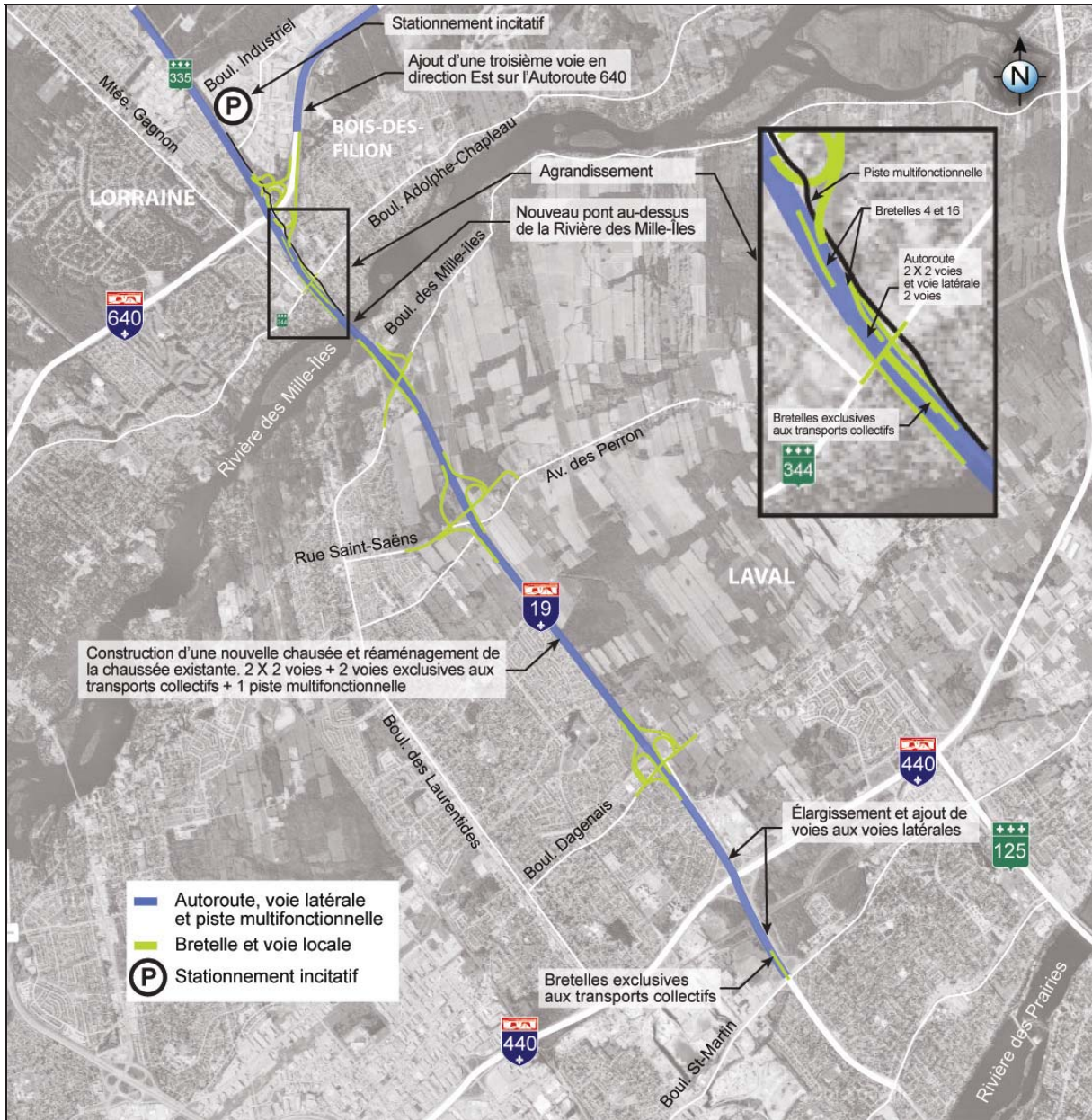
Figure 3 Vue générale du projet de parachèvement de l'autoroute 19 avec voie réservée au transport collectif dans chaque direction
