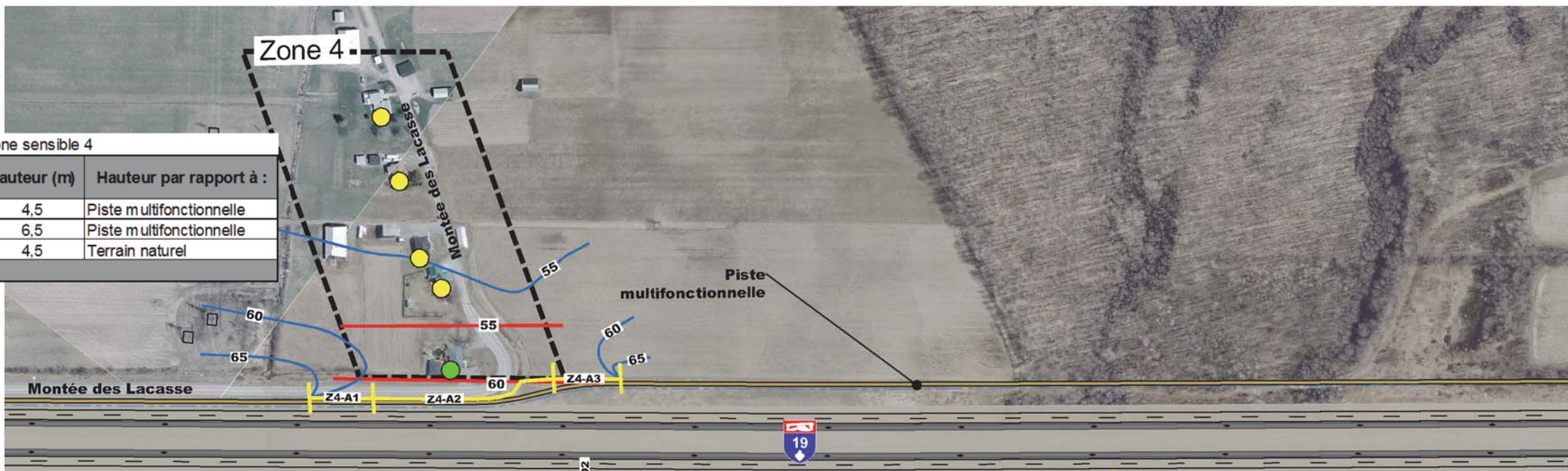
Écrans antibruit proposés pour la zone sensible 3 (partie nord)
