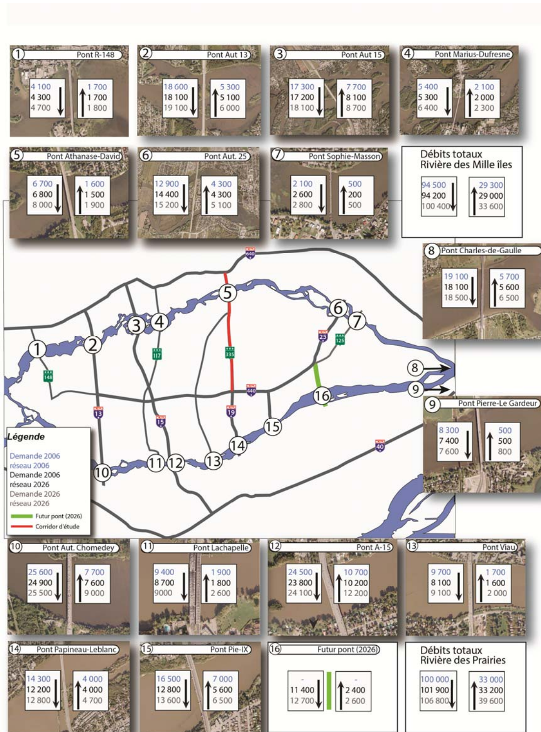
Figure 3-30 Débits sur les ponts autour de l'île Jésus, période de pointe du matin, 2006-2026
