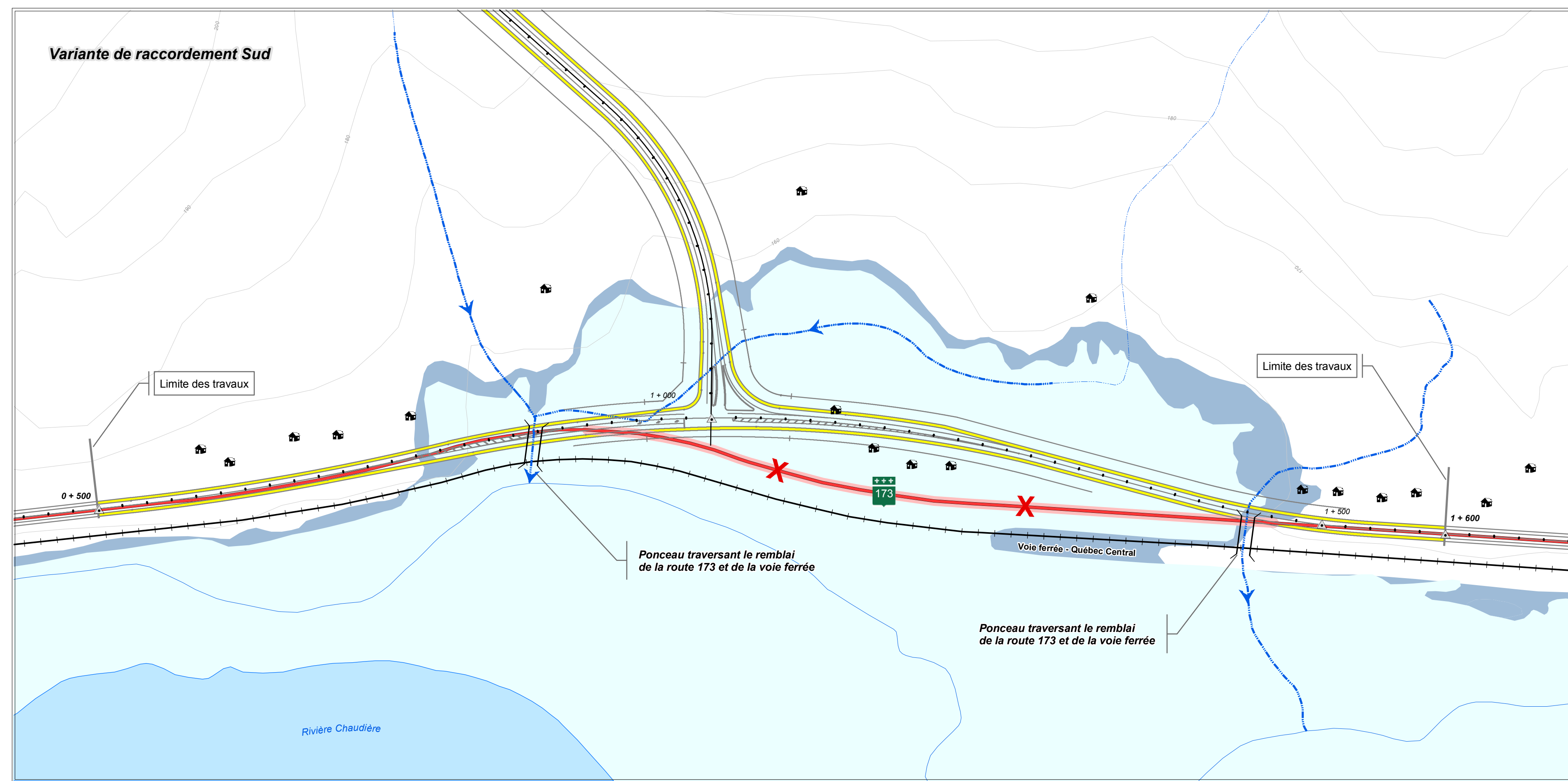
Figure 4 Nouvelle géométrie de la route 173 à la hauteur de son intersection avec le raccordement Sud (variante A)
