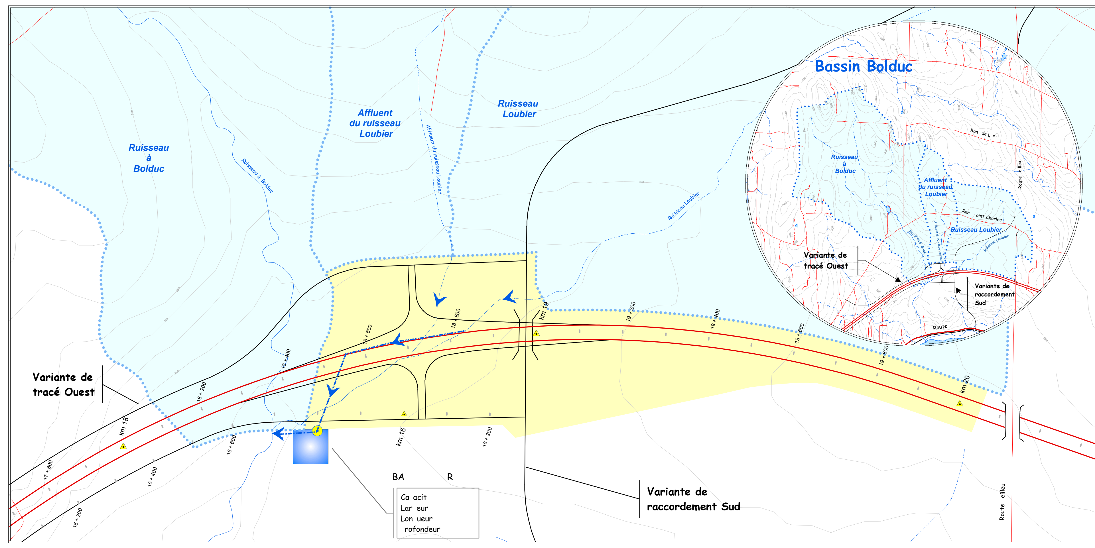
Figure 3 Travaux remédiateurs : rétention sur le bassin Bolduc avec contribution des fossés, tracé Ouest
