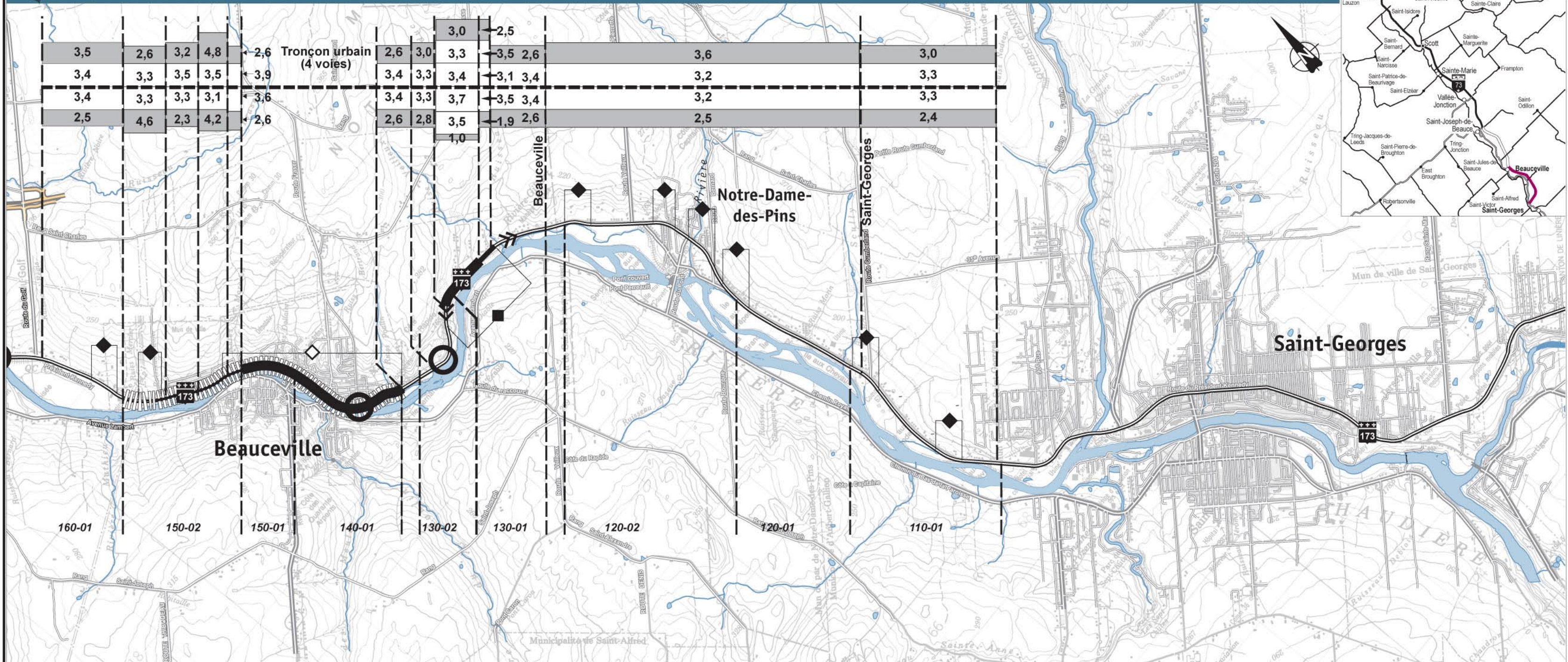
FIGURE 2.2 Caractéristiques géométriques et déficiences de la route 173 entre Beauceville et Saint-Georges
