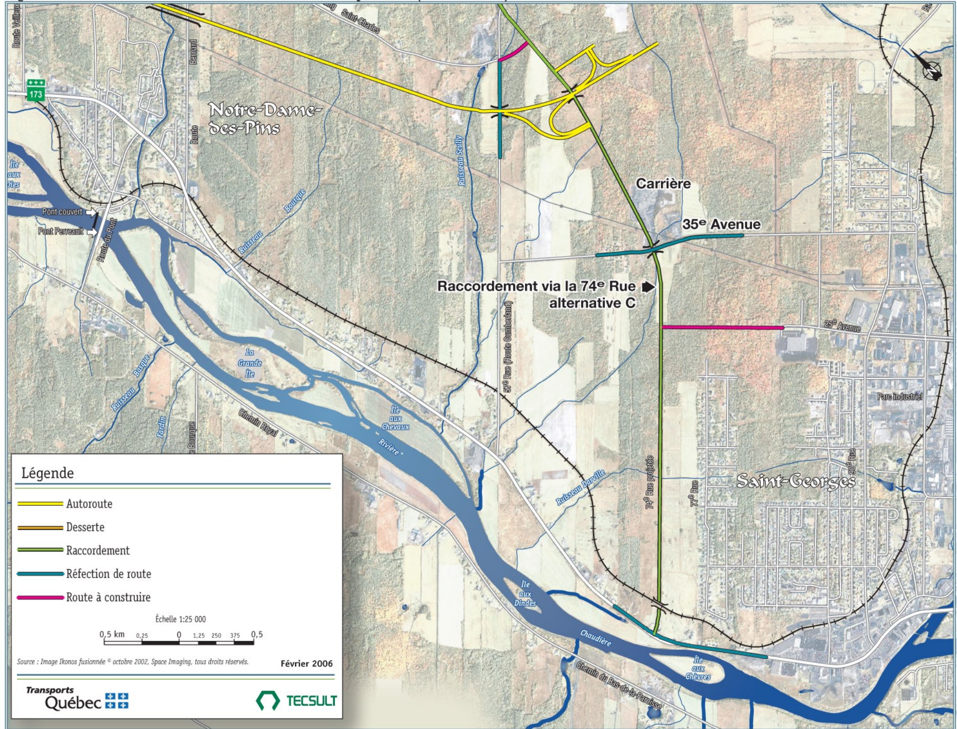
Figure 5.5 : Variante de raccordement via la 74 e Rue optimisée (alternative C)
