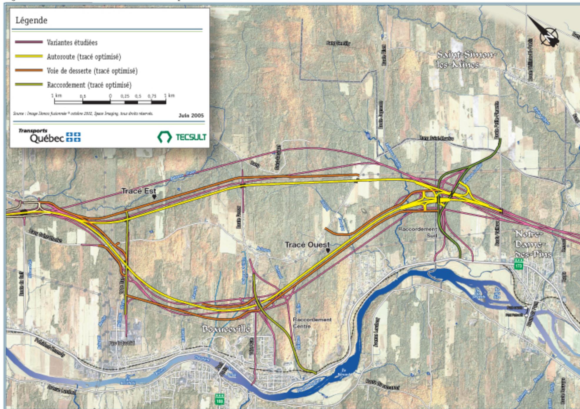
Figure 5.2 : Variantes successives et tracés optimisés
