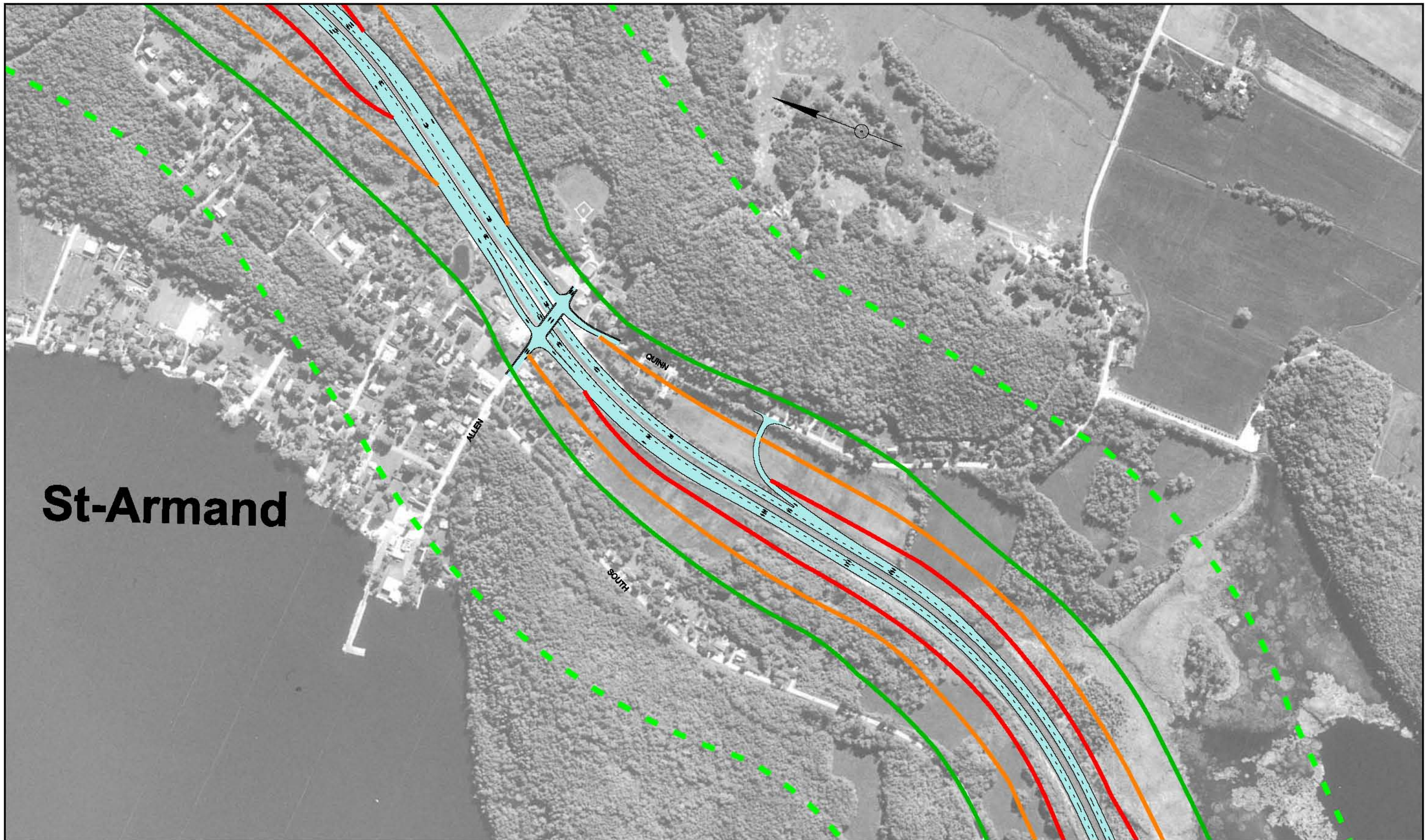
Groupe Conseil Génivar Figure 32 : Climat sonore projeté (2021) - secteur St-Armand (suite 2)
