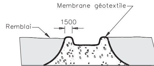
COUPE C-C
