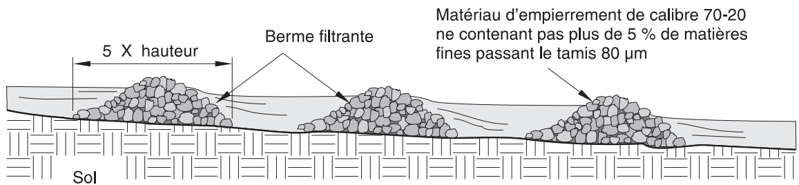
Figure 9.5-4 Trappe à sédiments et berme filtrante érigées dans un fossé routier
