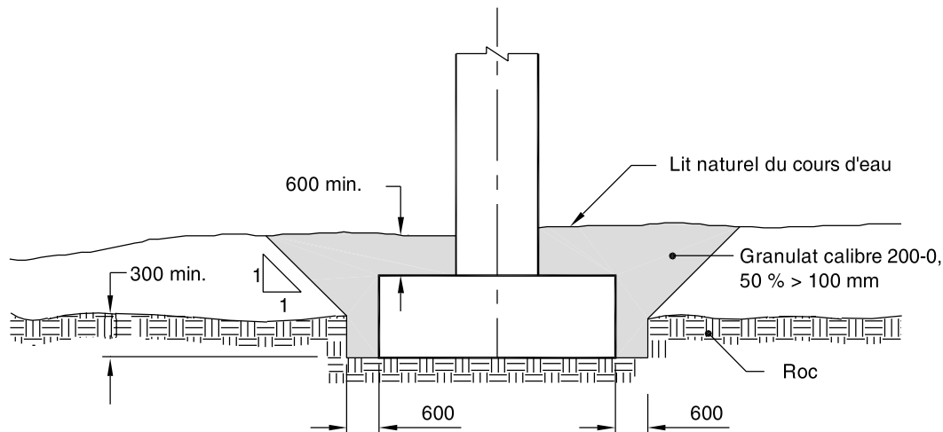
Figure 2.3–8 Pile en rivière, confinement d'une semelle sur roc
