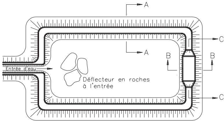
Bassin de sédimentation
