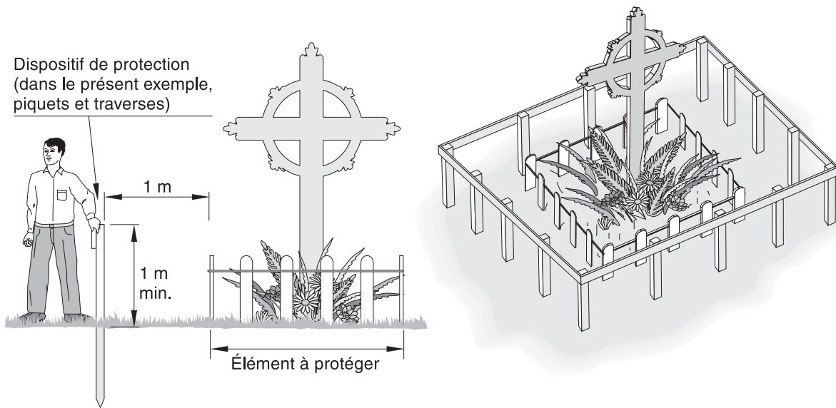
Figure 9.9-1 Protection d'un élément durant la construction
