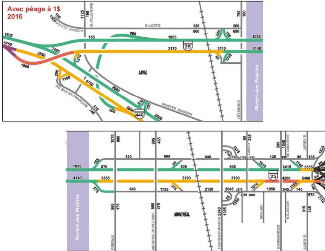
Fig. 2.3 - Débits et niveaux de service (2016, heure de pointe du matin)
