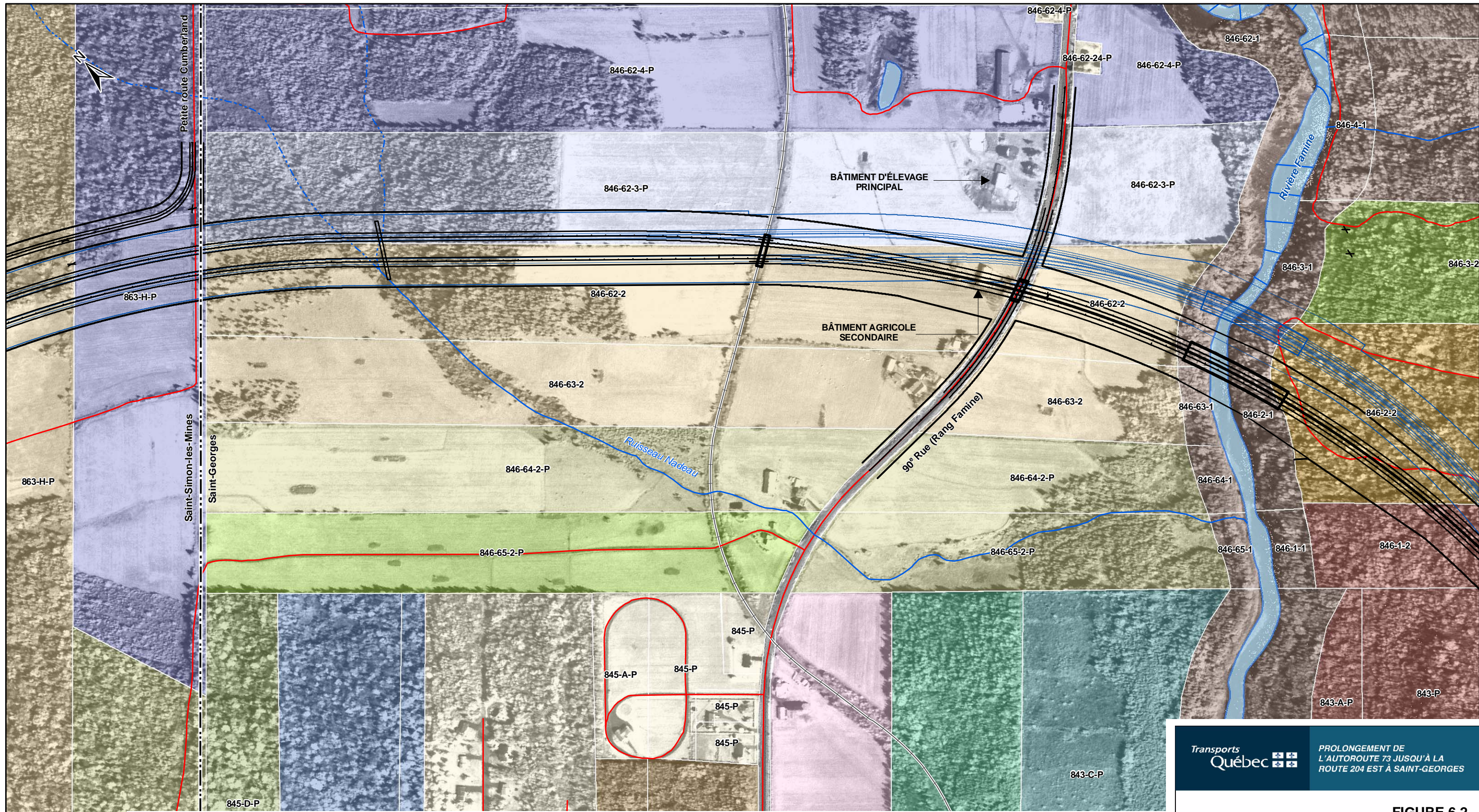
FIGURE 6.2 Optimisation du tracé dans le secteur de la 90 e Rue
