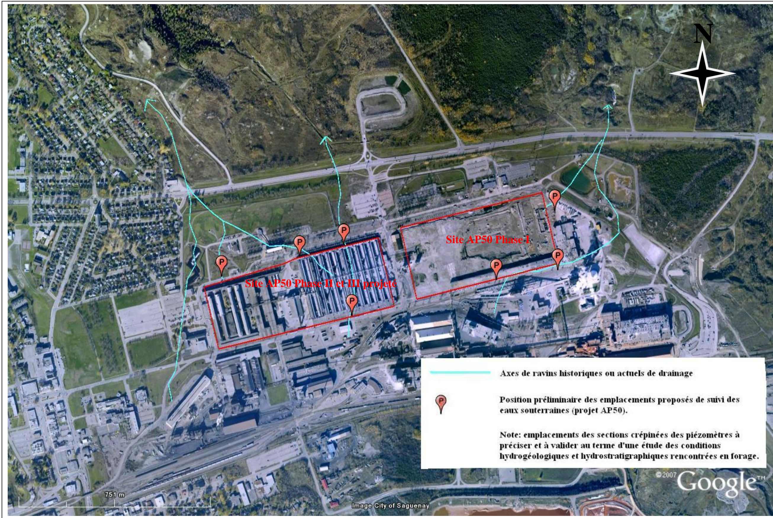
Figure E.1 : Position préliminaire des emplacements proposés de suivi des eaux souterraines (Projet AP-50), Complexe Jonquière RTA.
