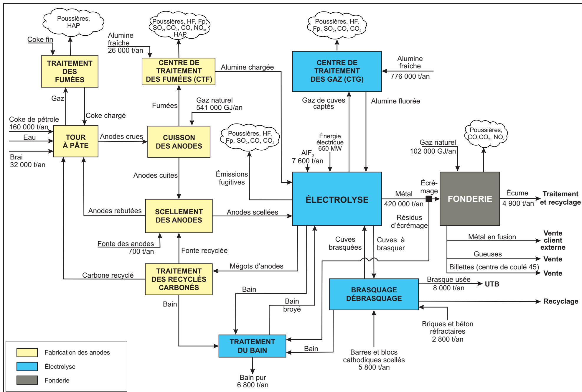
SCHÉMA DE PROCÉDÉ ET FLUX DE MATIÈRES - USINE AP50 JONQUIÈRE (420 000 t Al/an)
