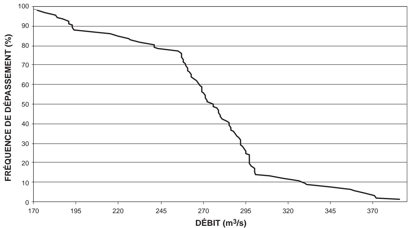
Figure A3.6 Courbe de débits classés pour des chutes brutes entre 4.50 m et 4.70 m au barrage des Quinze (92 jours de 1968 à 1990).
