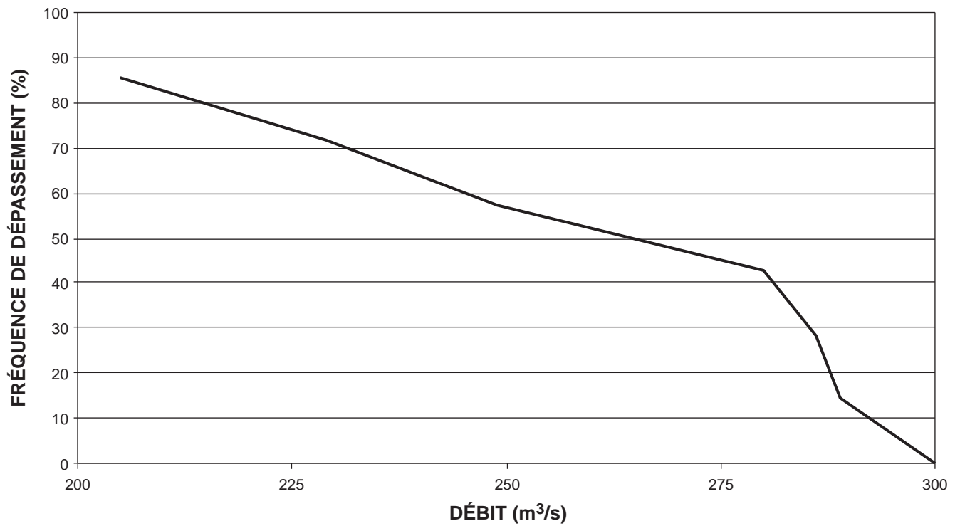
Figure A3.5 Courbe de débits classés pour des chutes brutes entre 4.40 m et 4.50 m au barrage des Quinze (7 jours de 1968 à 1990).
