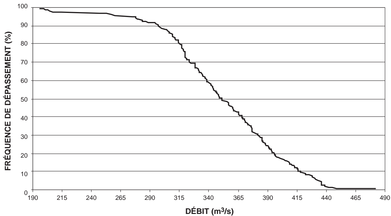
Figure A3.10 Courbe de débits classés pour des chutes brutes entre 5.30 m et 5.50 m au barrage des Quinze (259 jours de 1968 à 1990).
