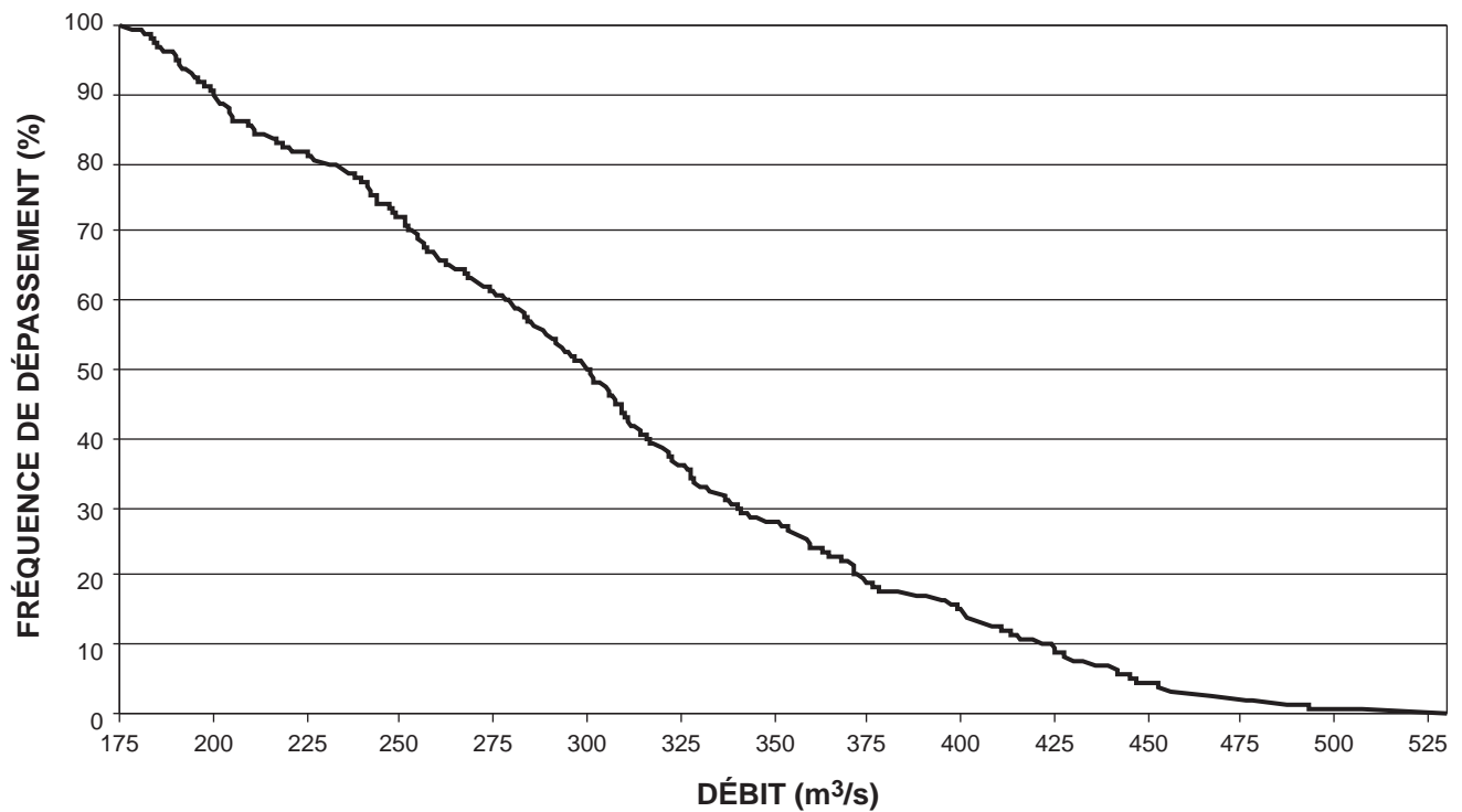
Figure A3.8 Courbe de débits classés pour des chutes brutes entre 4.90 m et 5.10 m au barrage des Quinze (327 jours de 1968 à 1990).
