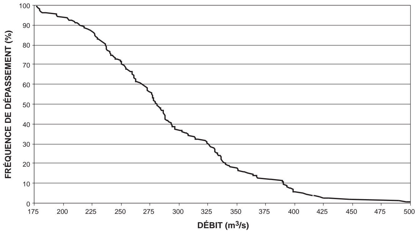
Figure A3.7 Courbe de débits classés pour des chutes brutes entre 4.70 m et 4.90 m au barrage des Quinze (219 jours de 1968 à 1990).
