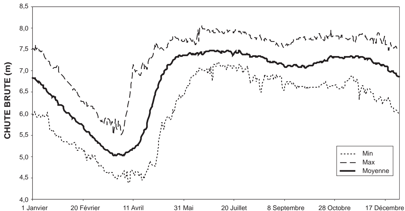
Figure A3.4 Évolution journalière de la chute brute au barrage des Quinze - courbe enveloppe et tendance moyenne (1967 à 1990).
