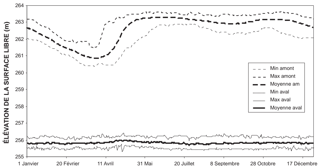
Figure A3.3 Évolution journalière de l'élévation de la surface libre à l'amont et à l'aval du barrage des Quinze - courbe enveloppe et tendance moyenne (1967 à 1990).
