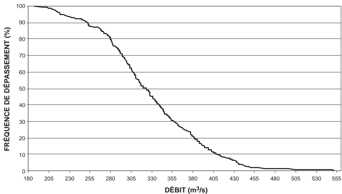
Figure A3.9 Courbe de débits classés pour des chutes brutes entre 5.10 m et 5.30 m au barrage des Quinze (378 jours de 1968 à 1990).
