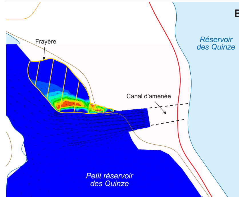
Fraysère aménagée – débit turbiné de 410 m 3 /s, centrale en fonction + 10 m 3 /s débit évacué – Indice global de la qualité
