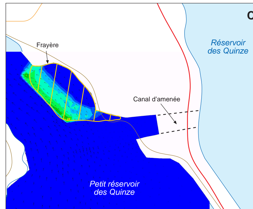
Fraysère aménagée – débit évacué de 420 m 3 /s – Centrale en arrêt – Indice global de la qualité
