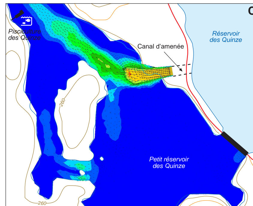
Débit de 420 m 3 /s – Centrale en fonction
