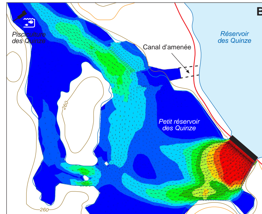
Débit de 420 m 3 /s – Centrale en arrêt
