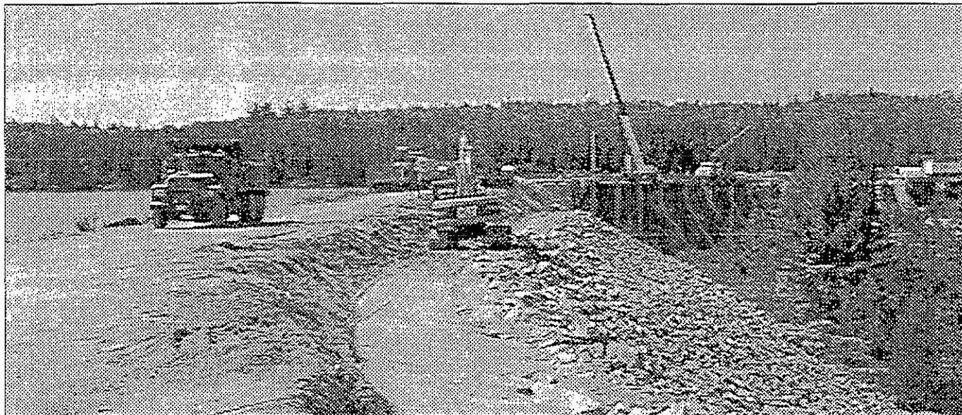
Début septembre 2002, les travaux de rehaussement du barrage en enrochement de l'évacuateur des Rapides-des-Quinze vont bon train.
