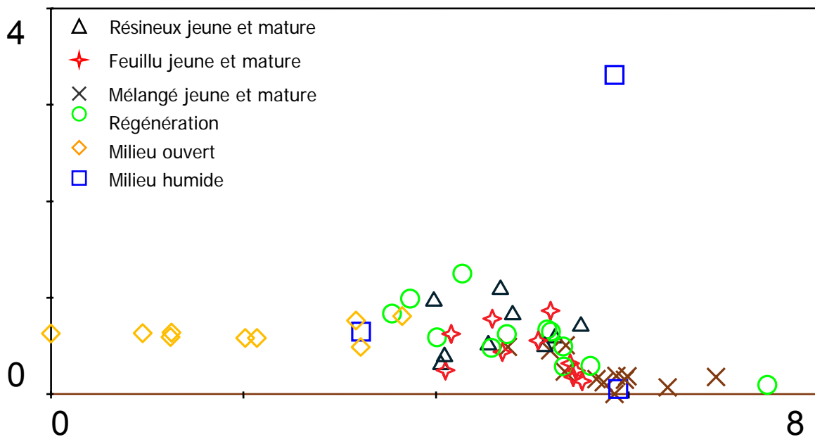
Figure 3 Répartition des stations de chaque habitat selon une analyse d'ordination de type DCA basée sur les oiseaux recensés lors des points d'écoute DRL effectués au printemps 2003 (chaque point équivaut à une station)
