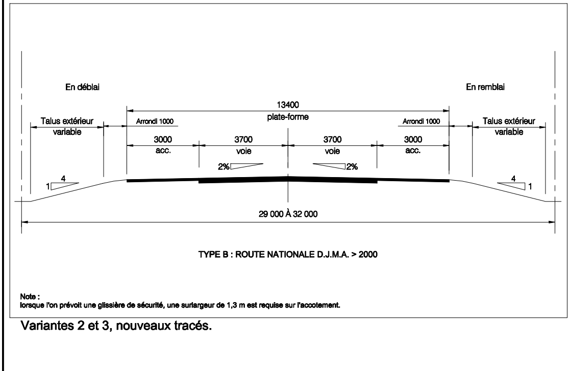
Figure 5.1 Sections-types des variantes du réaménagement de la route 138 à Sainte-Anne-de-Portneuf
