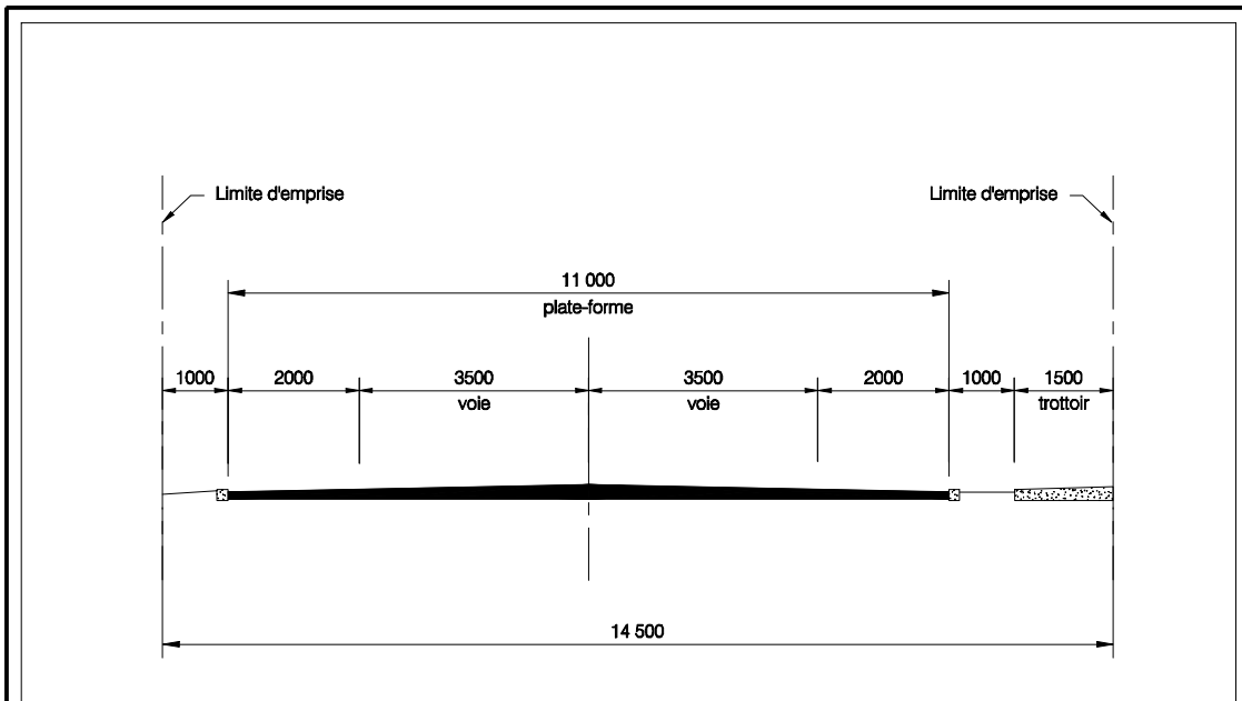
Variante 1, tracé actuel.
