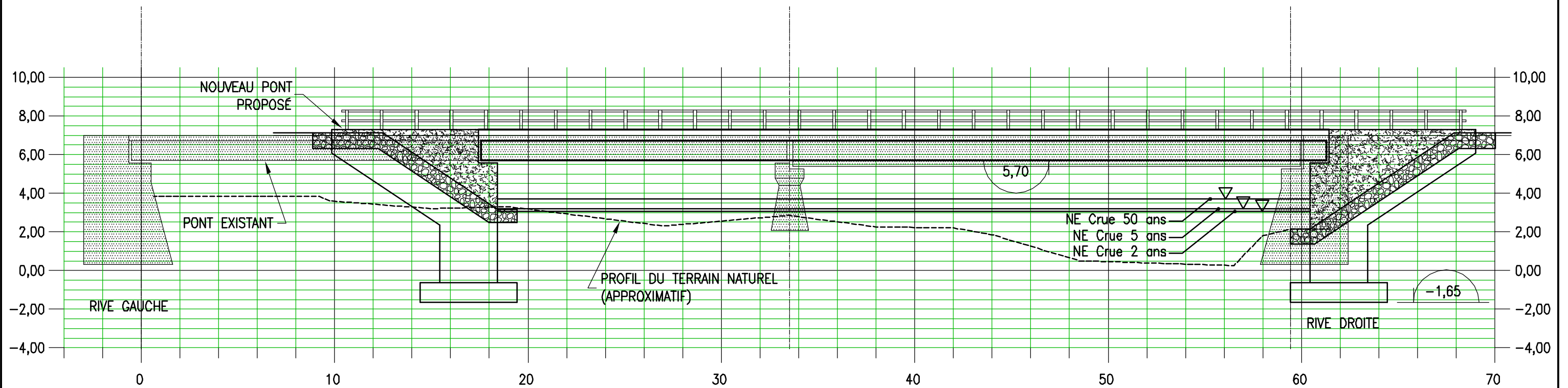
PROFIL TRANSVERSAL 1:200
