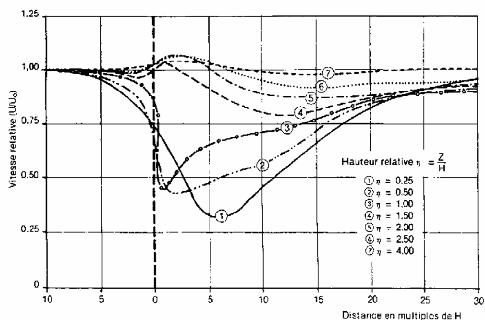
Figure 4- Influence d'un brise-vent perméable ( 0,45 < \phi < 0,55 ) et H = 2,2 m) constitué par une claie de roseaux sur la vitesse relative du vent à différents niveaux (d'après Nagéli, 1953 dans Guyot, 1989).
