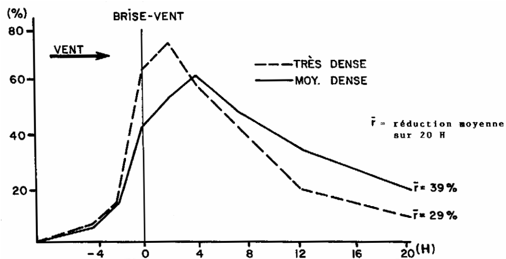
Figure 2- Réduction de la vitesse du vent (en % de la vitesse mesurée en zone ouverte) à différentes distances de brise-vent constitués de claies de roseaux très denses et moyennement denses (d'après Nagëli dans Guyot, 1977).
