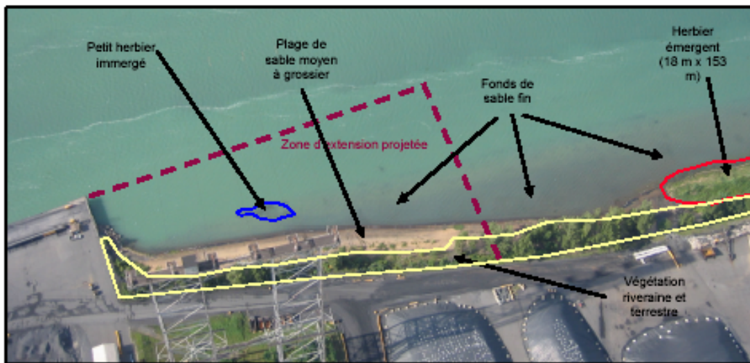
Photo 1: Vue aérienne de la zone de remblai projeté
