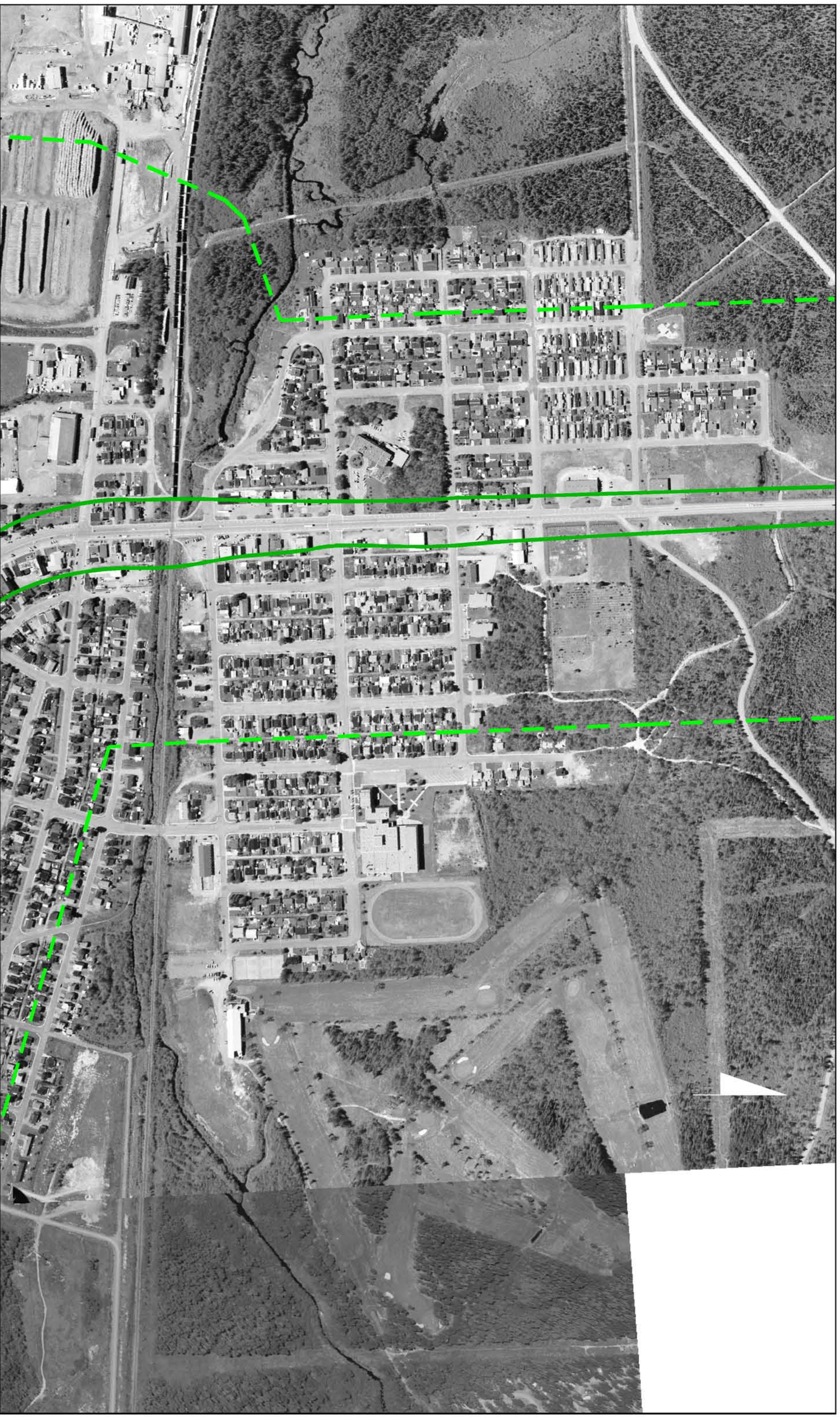
Figure 10 : Climat sonore simulé actuel le long de la route 117
