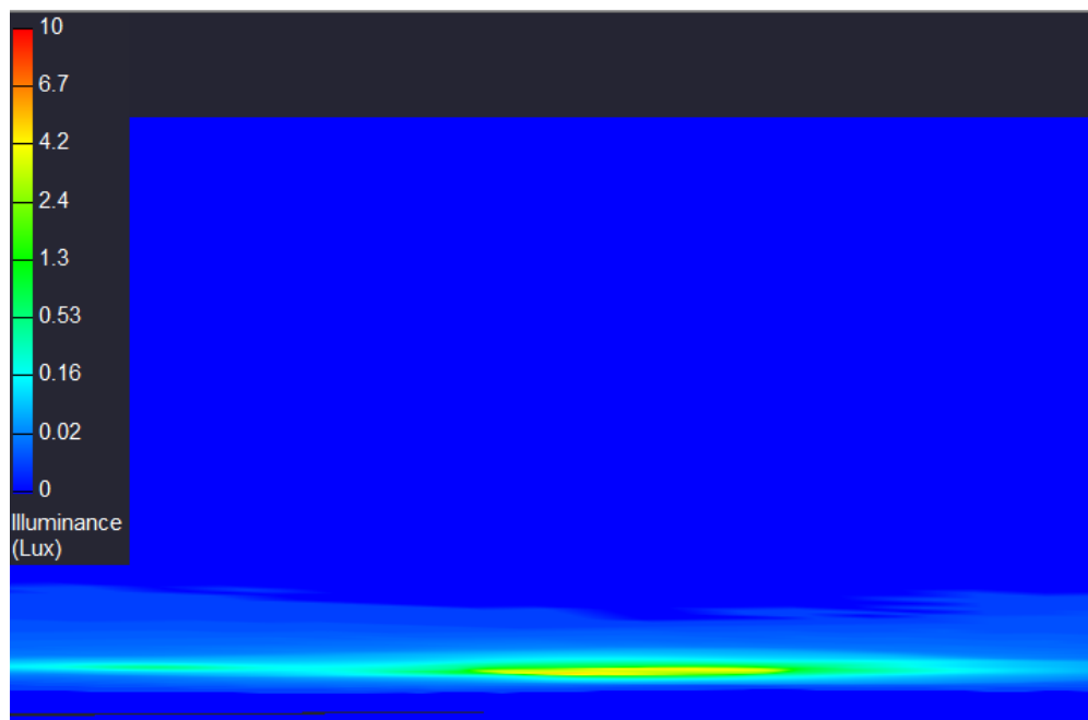
Figure 7 Charte de couleur montrant les niveaux d'éclairage des futures installations à partir du secteur des chalets du lac Bayeul à 100 m au-dessus du sol en hiver
