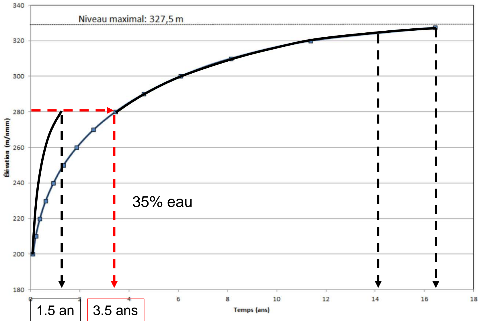
Mines Agnico-Eagle - projet Akasaba Ouest Courbe d'ennoiement de la fosse en fonction du temps
