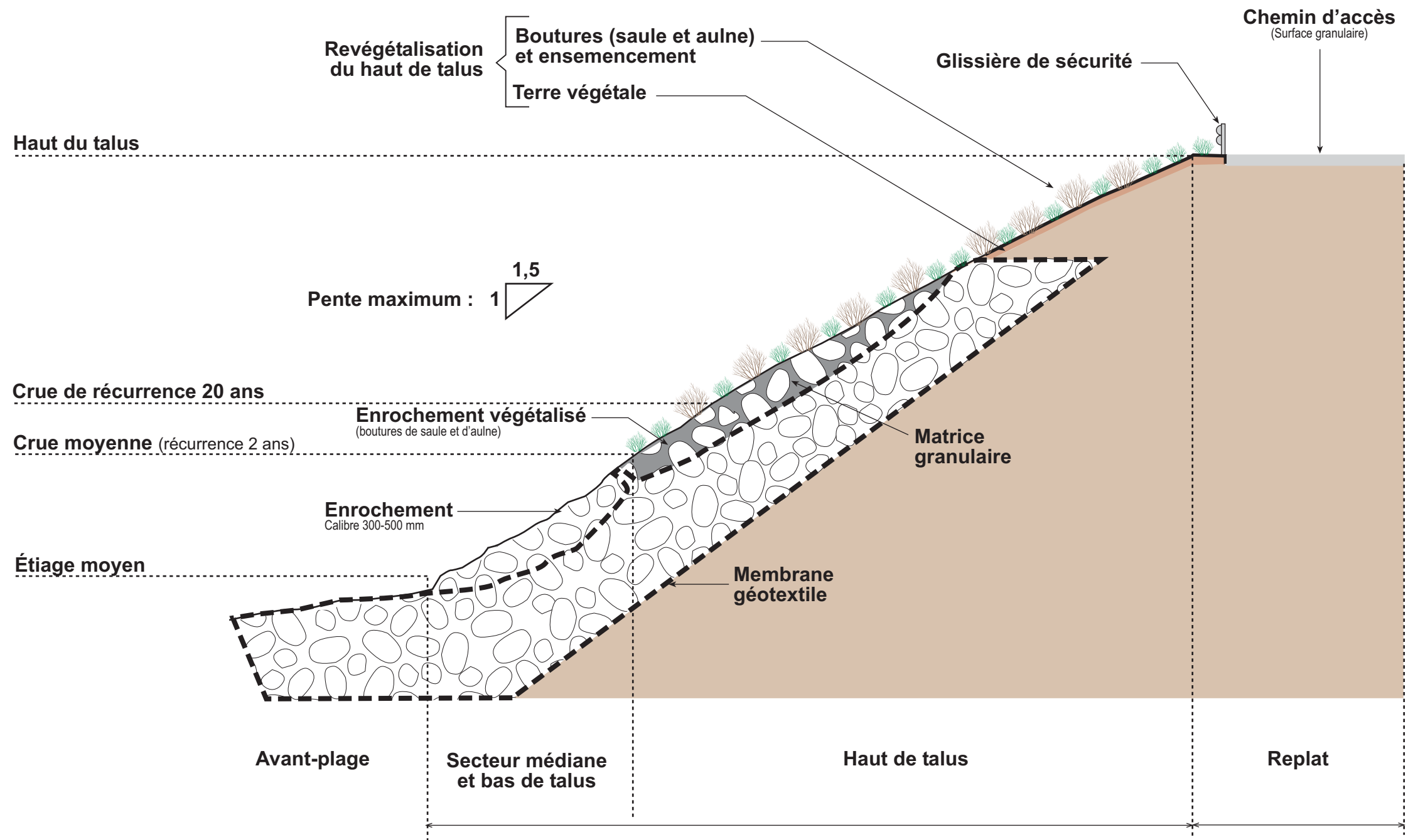
INNERGEX II IMPLANTATION D'UNE MINICENTRALE HYDROÉLECTRIQUE AU BARRAGE MATAWIN Figure 2-1 Végétalisation du perré du chemin d'accès - coupe type
