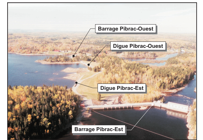
Barrages et digues Pibrac-Est et Pibrac-Ouest
