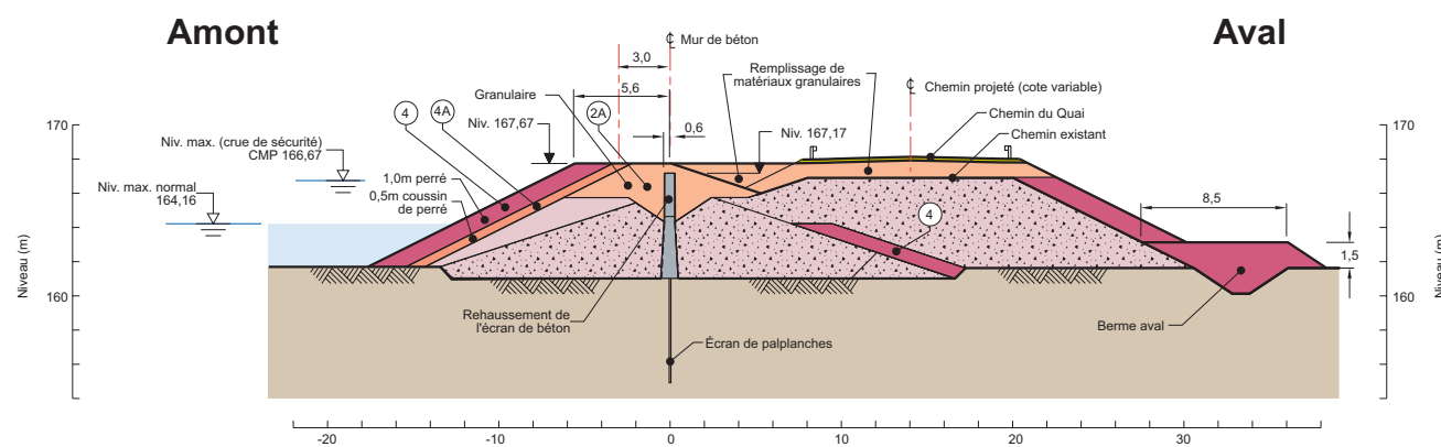
Coupe type Travaux de rehaussement et berme aval
