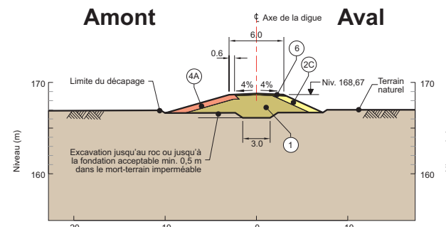
Coupe B-B - Digue du point bas n° 15
