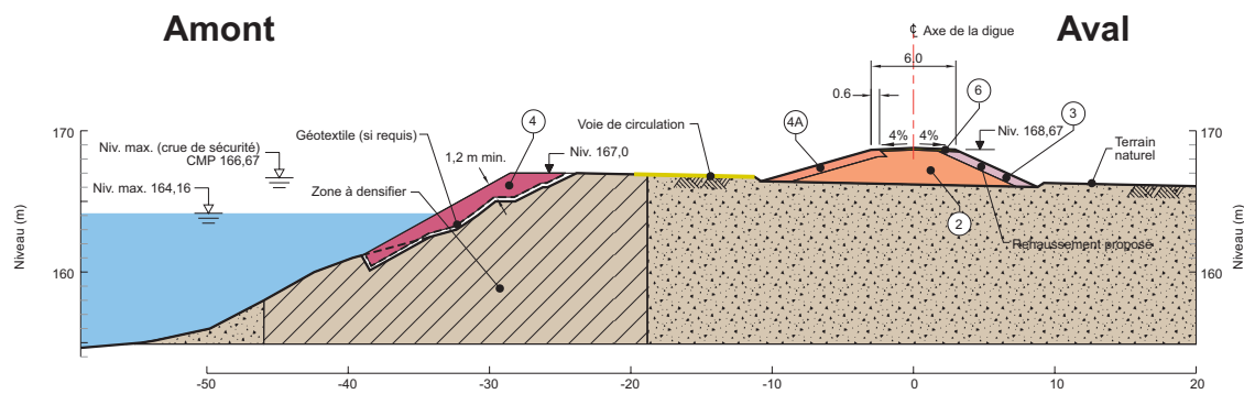
Coupe A-A - Digue Ouiqui
