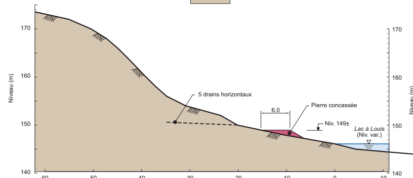
Coupe C-C - Protection du talus instable
