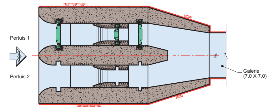
Coupe B-B
