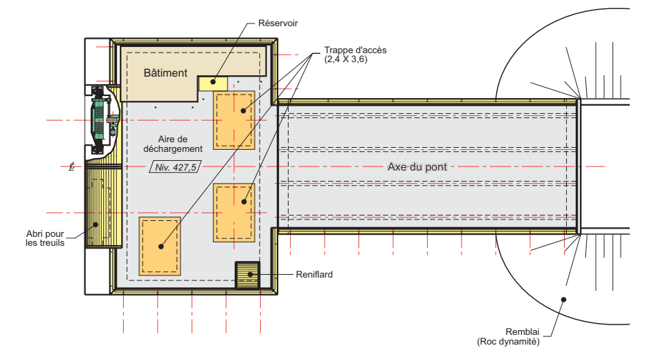
Coupe F-F
